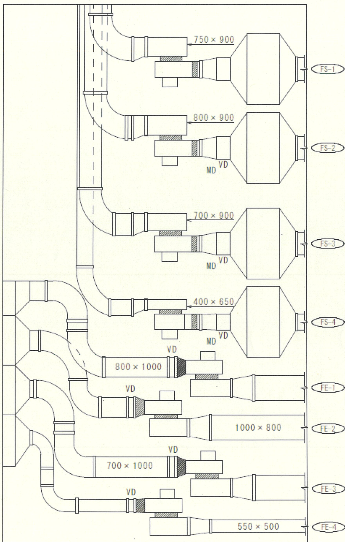
中2階ファン室廻り平面図
