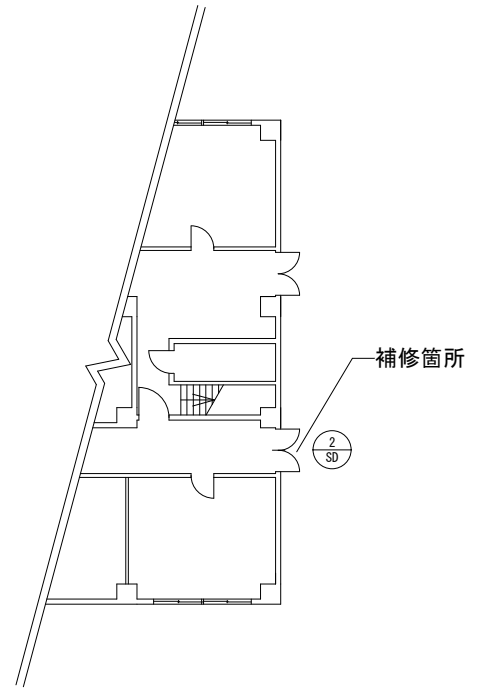
217号建物1階平面図 S = 1 / 300
