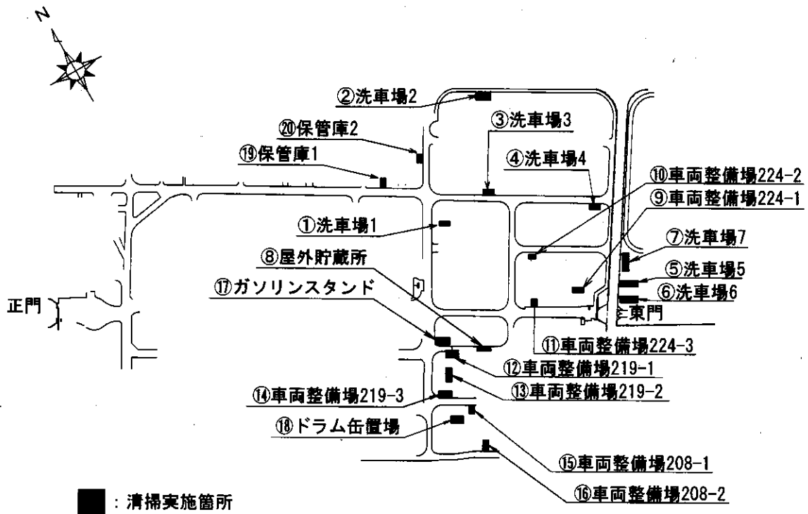
駐屯地配置図 S=1/5,000
