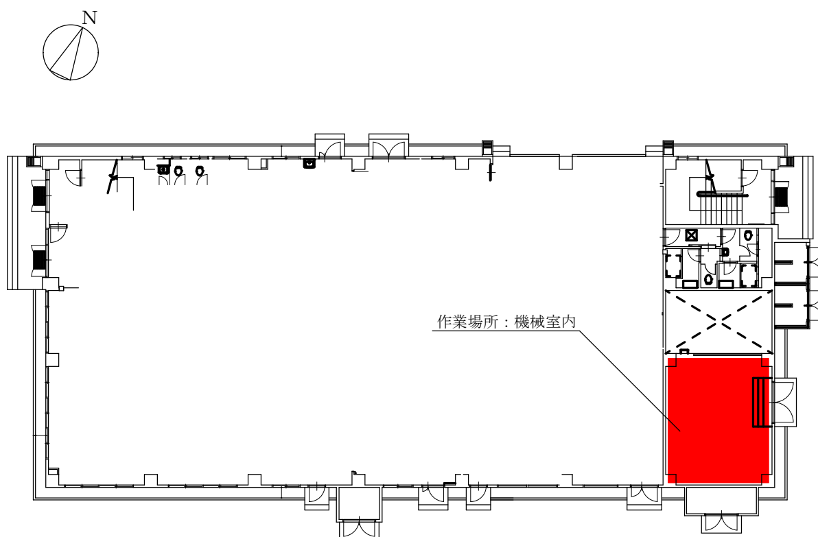
5 2 号 1 F 平面図 S=1:300
