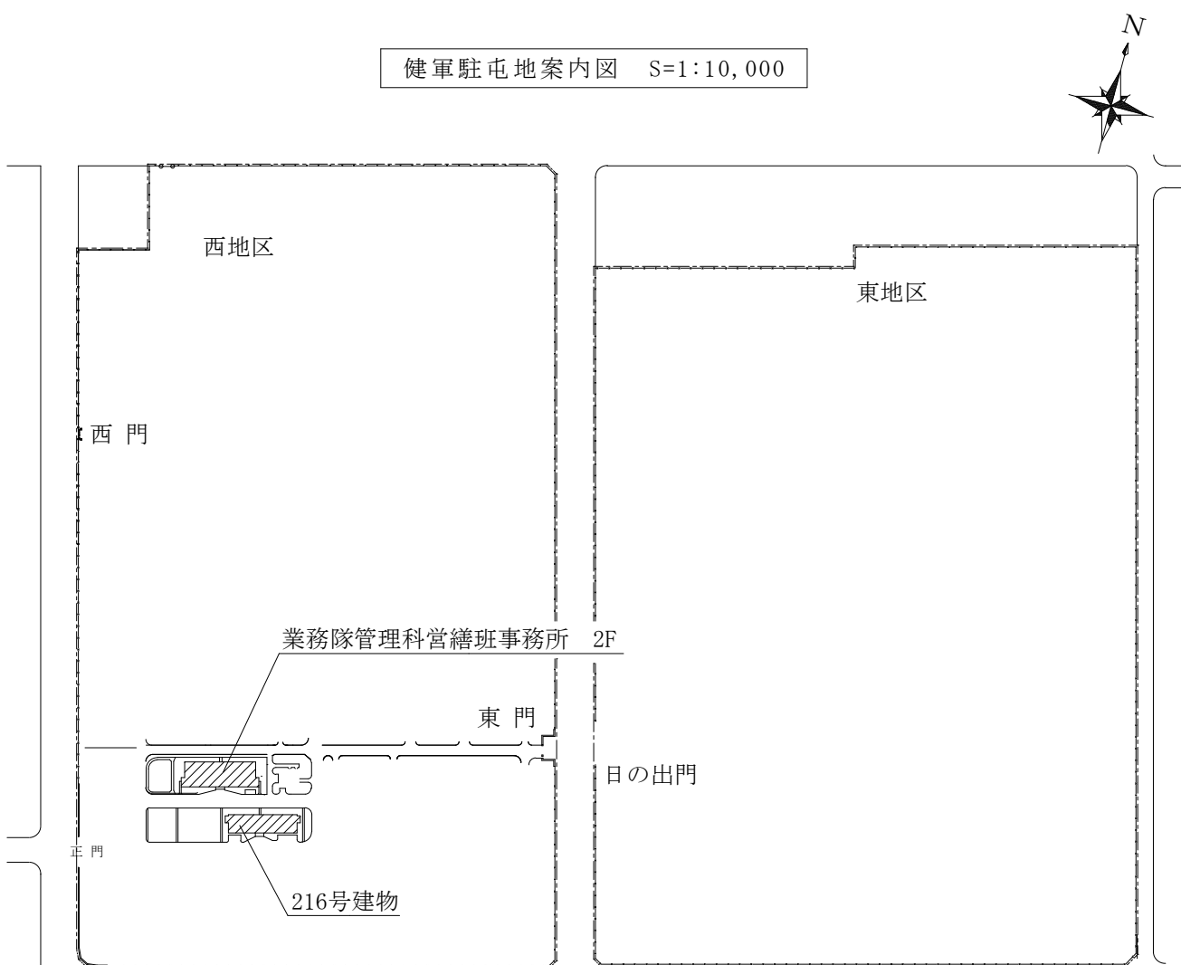
健軍駐屯地配置図 S=1:6,000
