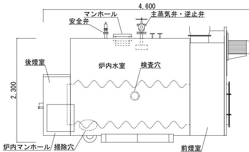
ボイラー内部図 S=1/50
