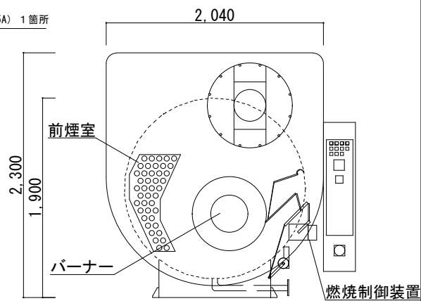
ボイラー正面図 S=1/50
