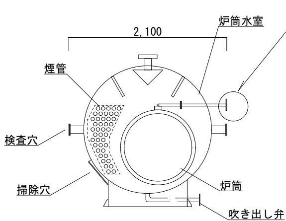
ボイラー内部図 S=1/50
