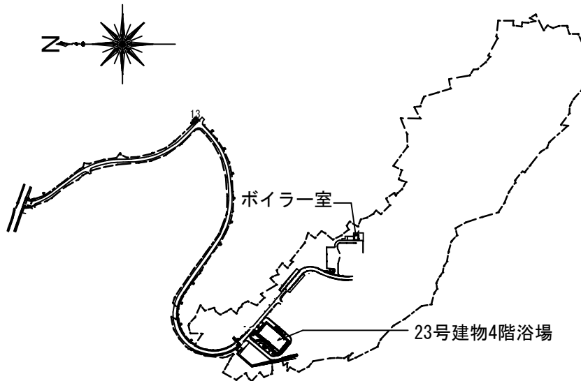
勝連分屯地配置図 S=1:X
