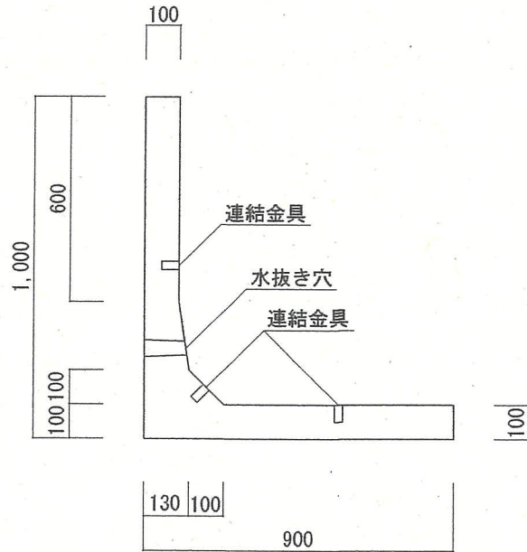
L型擁壁断面図 S=1/20
