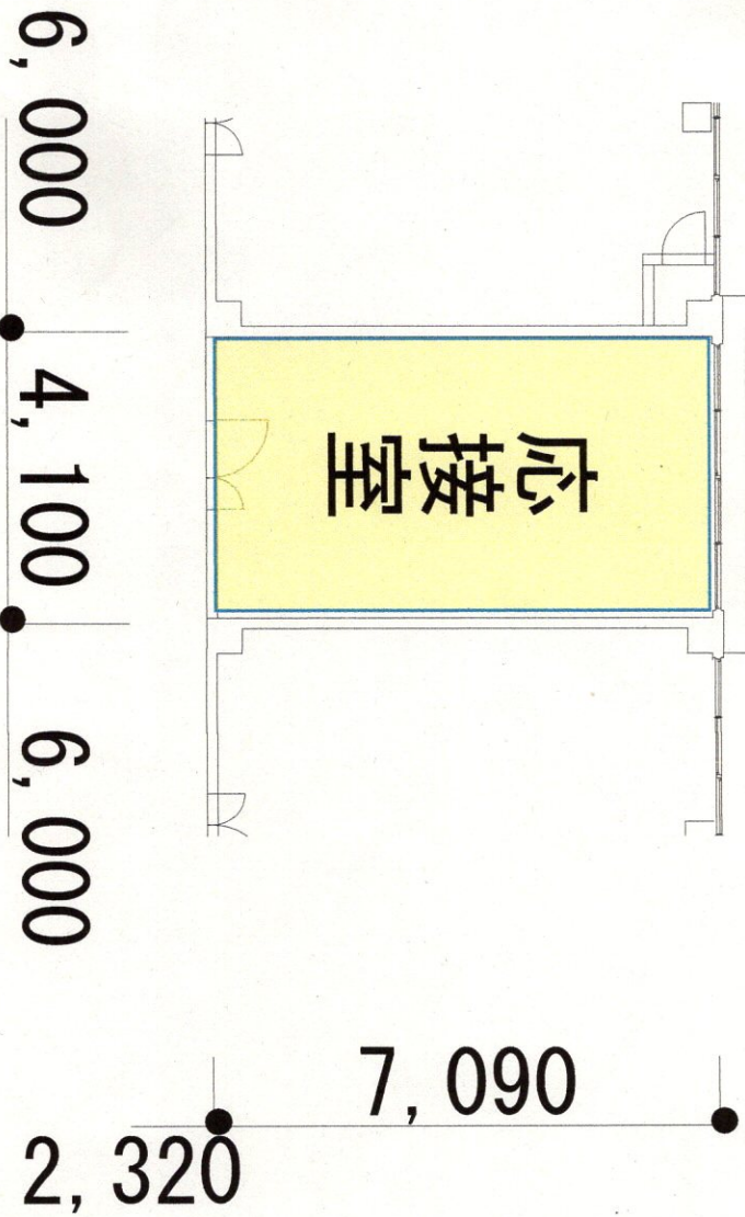
応接室拡大図
