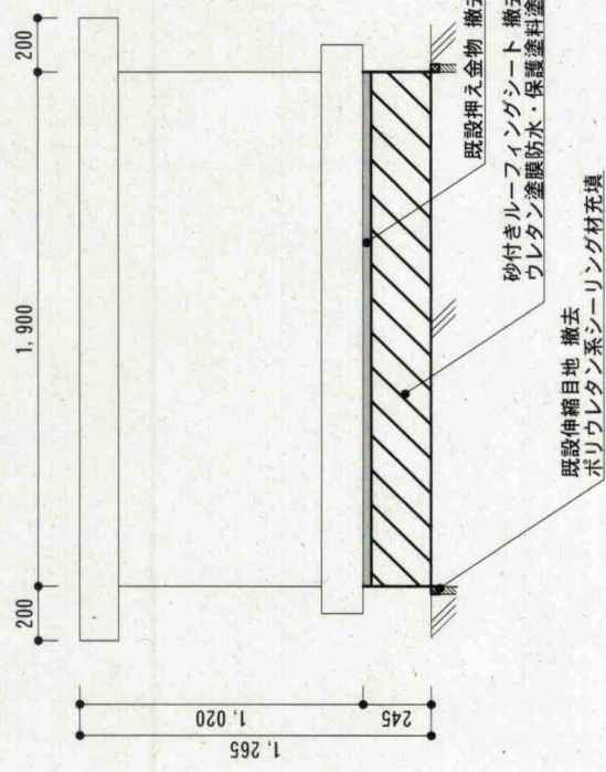
配管用ハト小屋立上り (大) 正面詳細図
