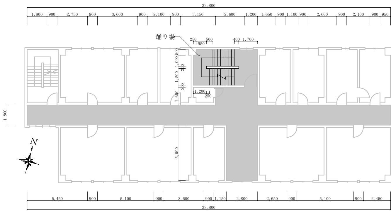
148号建物2F平面図 S=1/200
