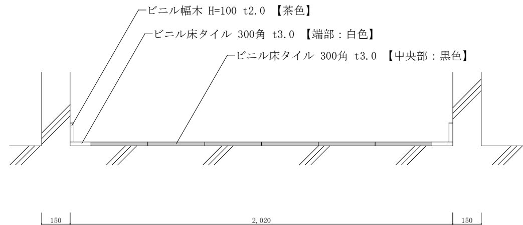
17号隊舎断面詳細図[標準] S=1/20
