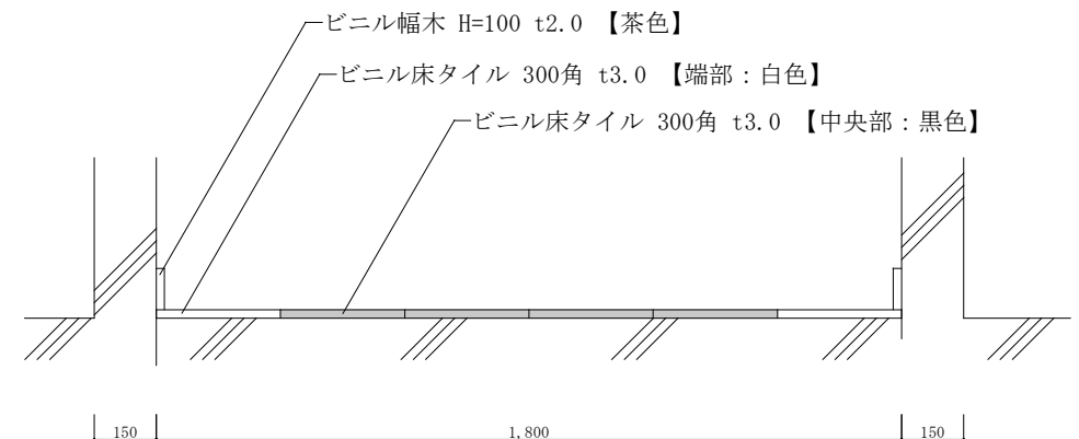
148号隊舎断面詳細図[標準] S=1/20
