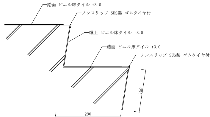
階段詳細図 [標準] S=1/10
