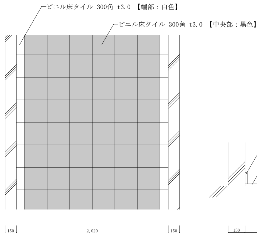
17号隊舎平面詳細図[標準] S=1/30
