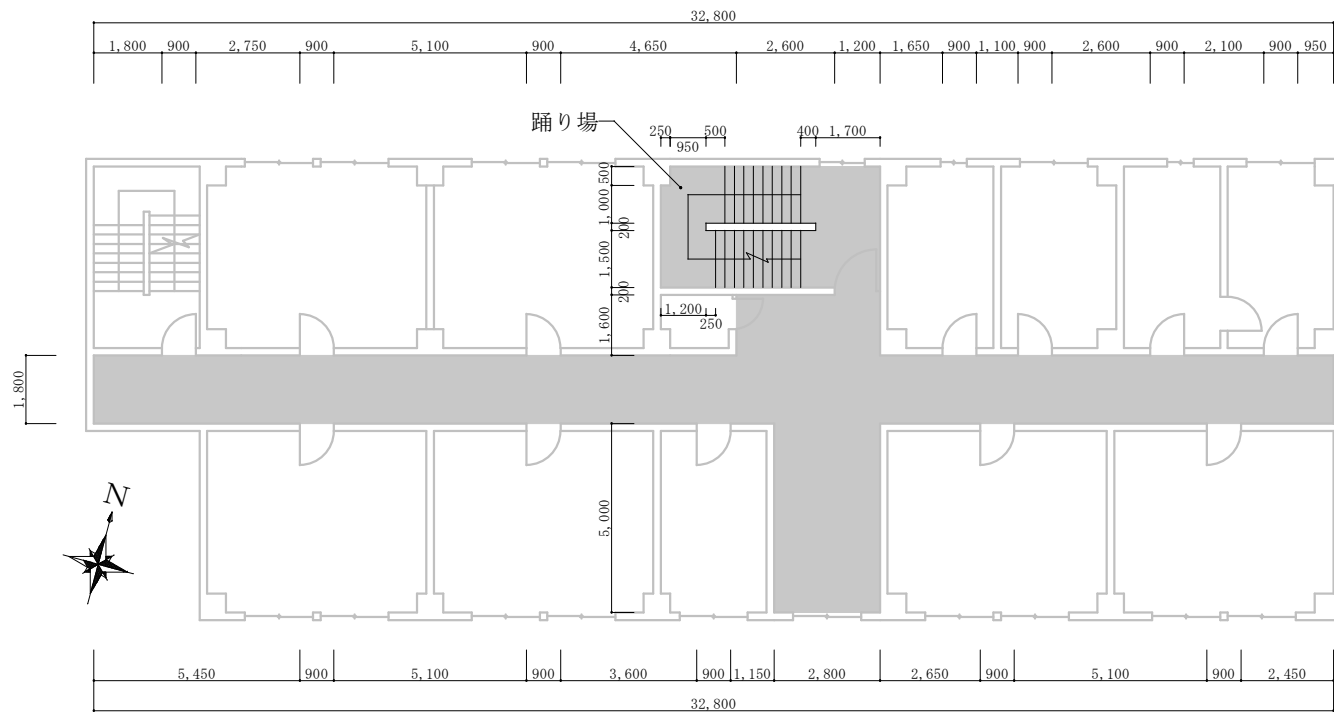
148号建物3F平面図 S=1/200
