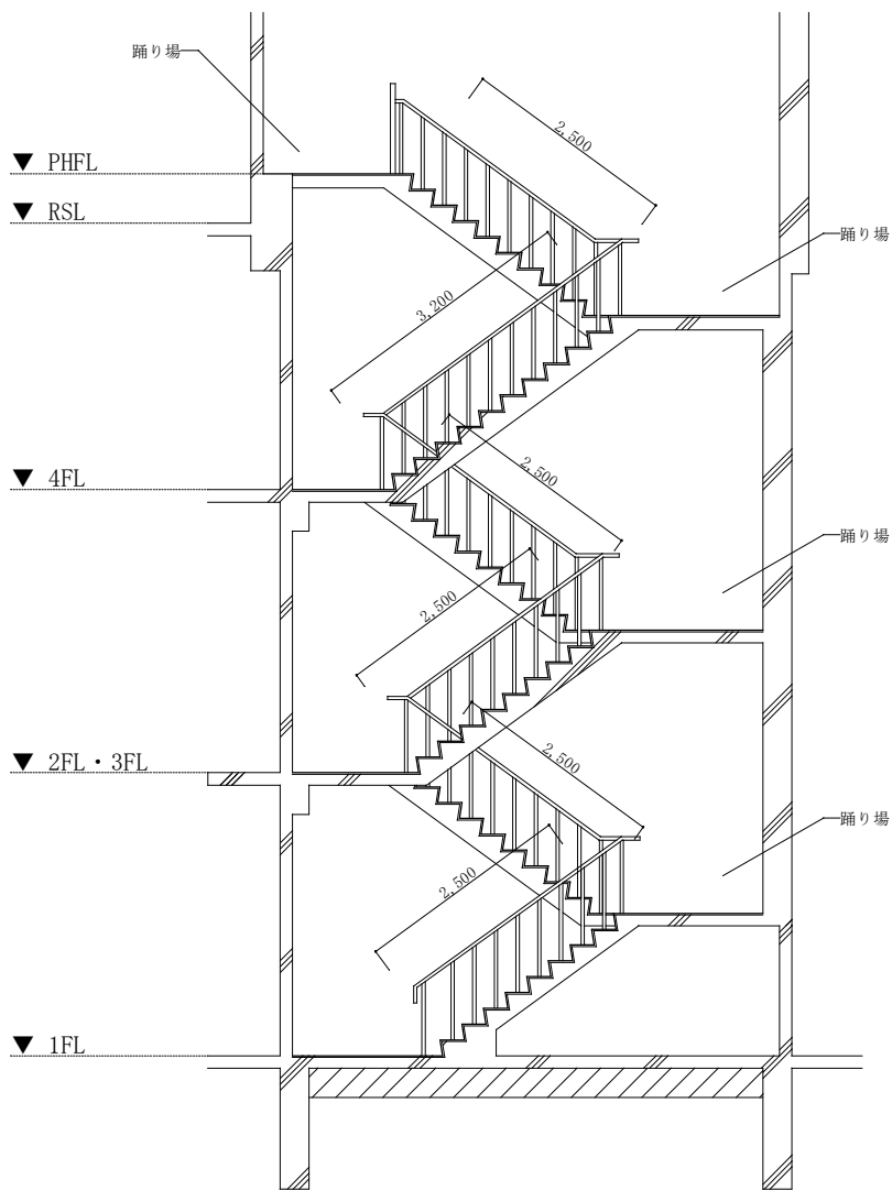
148号建物階段断面図 S=1/100
