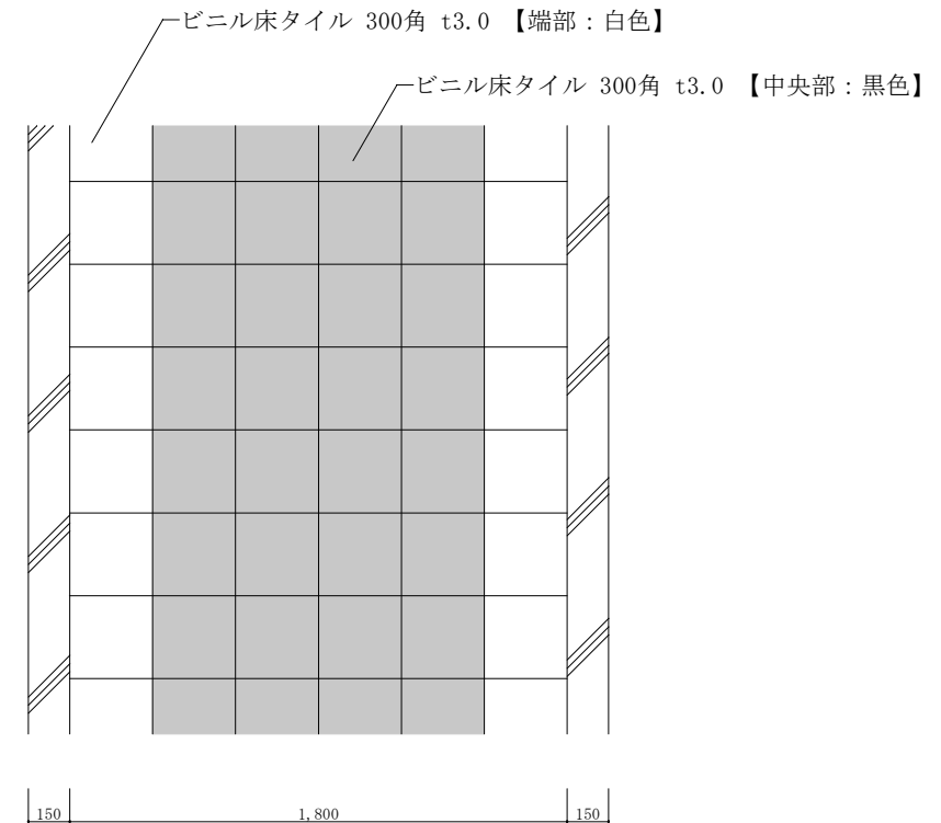
148号隊舎平面詳細図[標準] S=1/30
