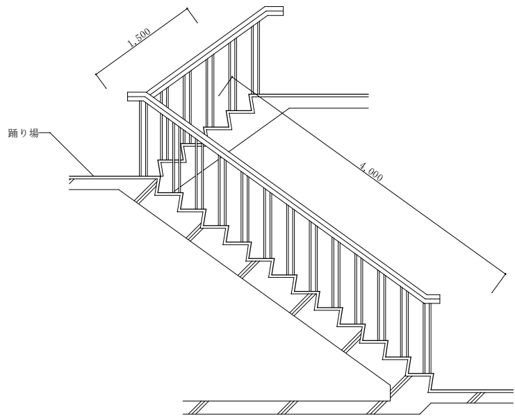
17号建物階段断面図 S=1/60
