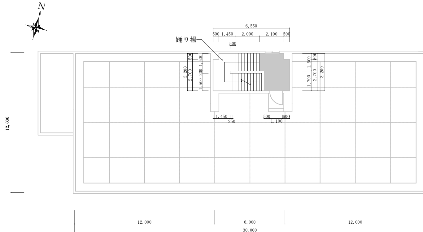
148号建物PH平面図 S=1/200 ■■■■ ・・・施工範囲を示す
