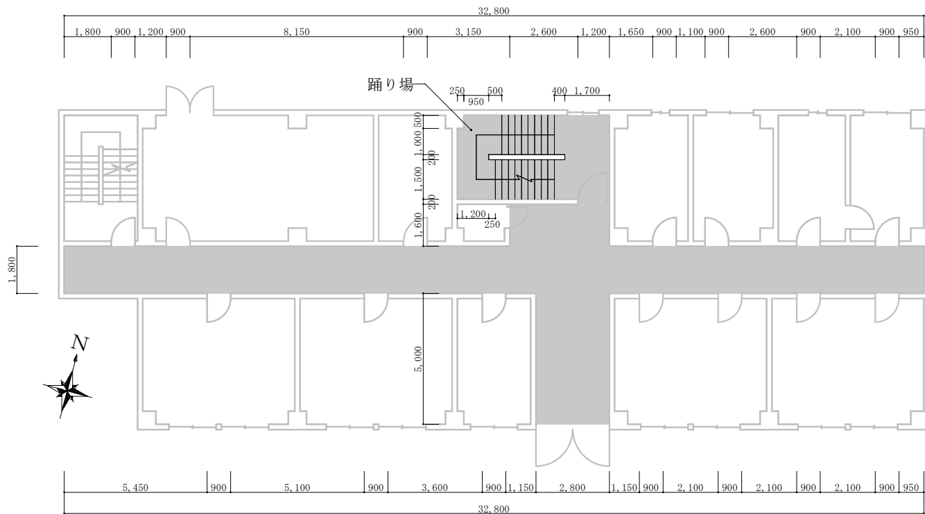
148号建物1F平面図 S=1/200
