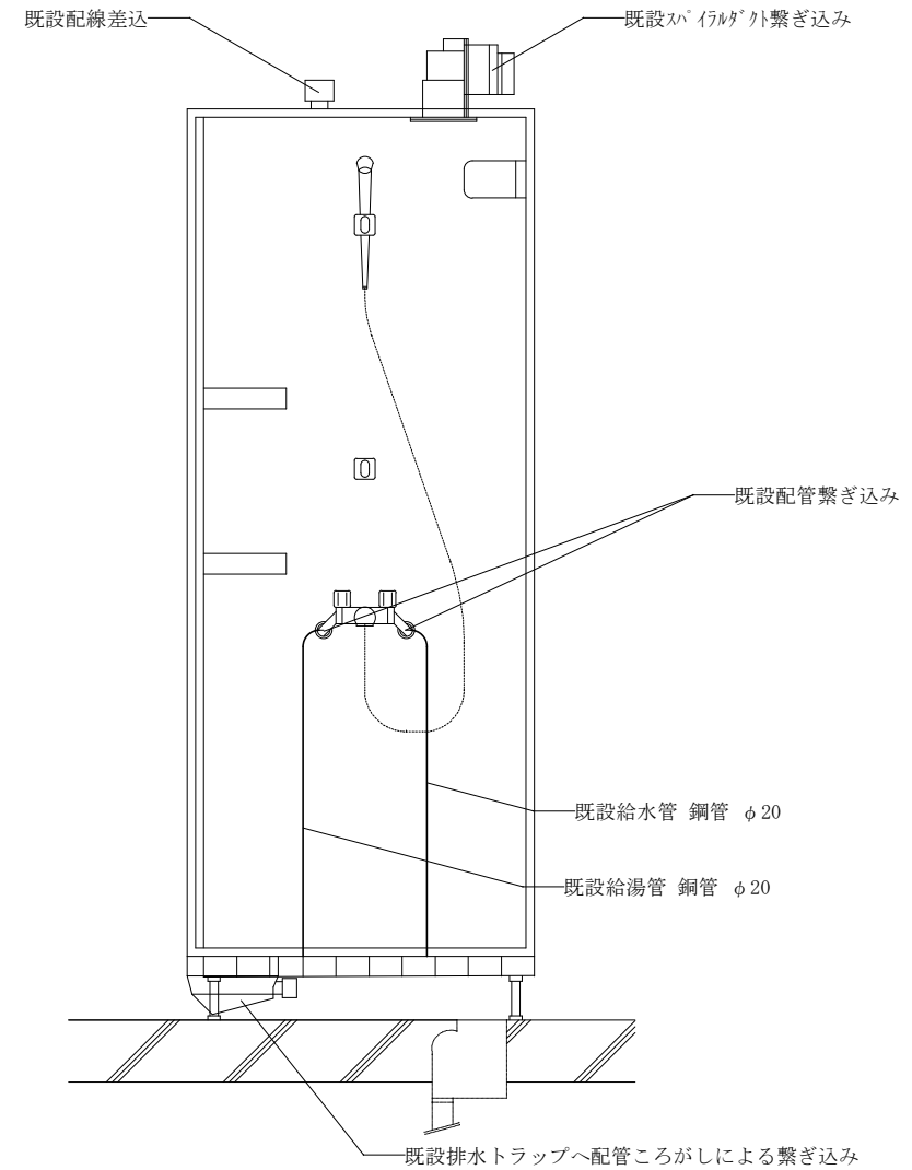
設備詳細図(新設) S=1/20
