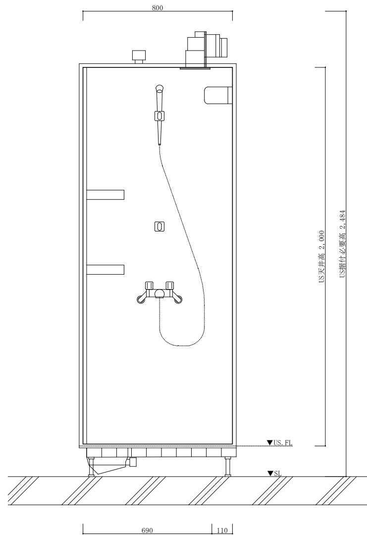
新設 U S 詳細図 (標準) S=1/20
