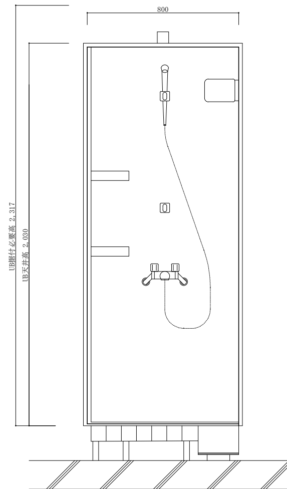
既設 U S 詳細図 (標準) S=1/20
