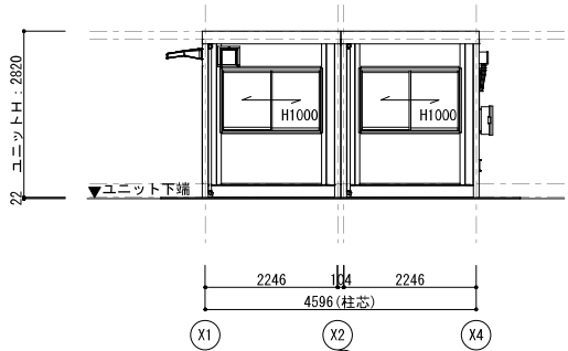
Y1通り立面図
