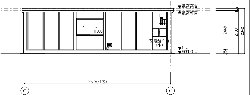
X4通り立面図
