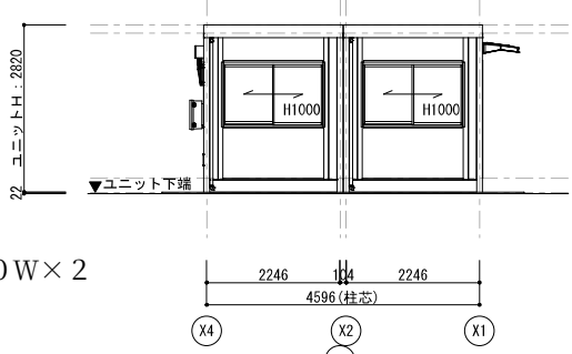
Y2通り立面図
