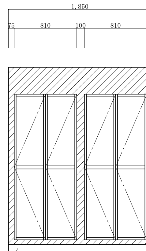
シャワー室D面展開図 S=1/30
