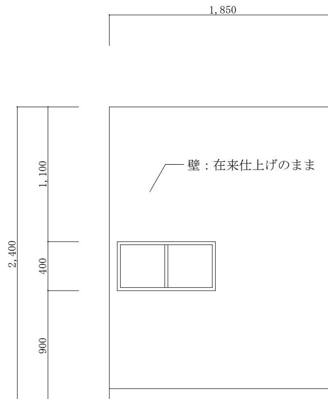
シャワー室B面展開図 S=1/30
