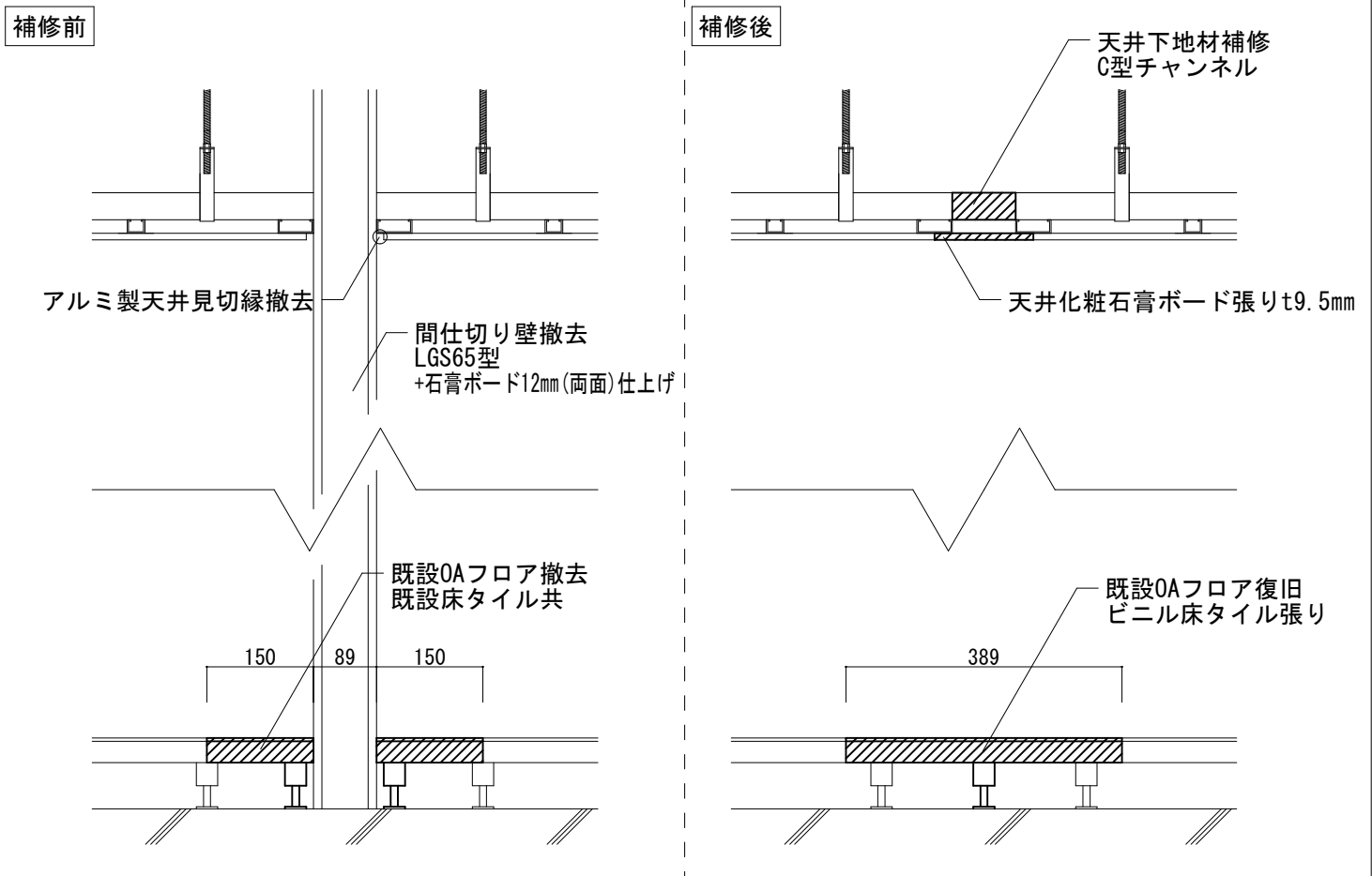
施工箇所④天井・床補修断面詳細図 (補修前・後) S=1/10
