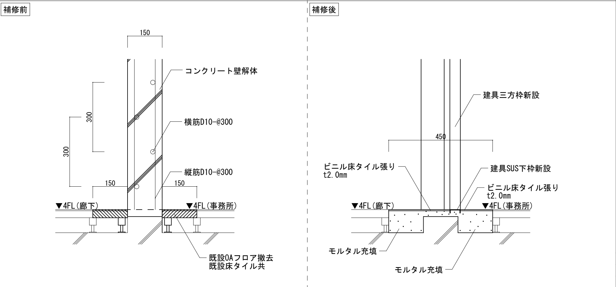
施工箇所⑦解体壁断面詳細図 S=1/10
