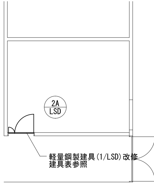
施工箇所③平面詳細図 S=1/100
