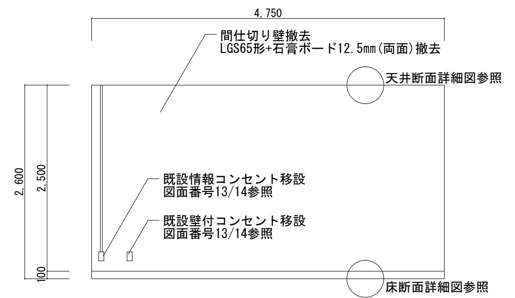
事務室④展開図D(撤去前) S=1/50
