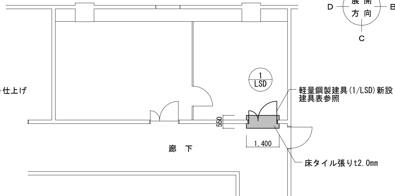
施工箇所②平面詳細図(改修後) S=1/100
