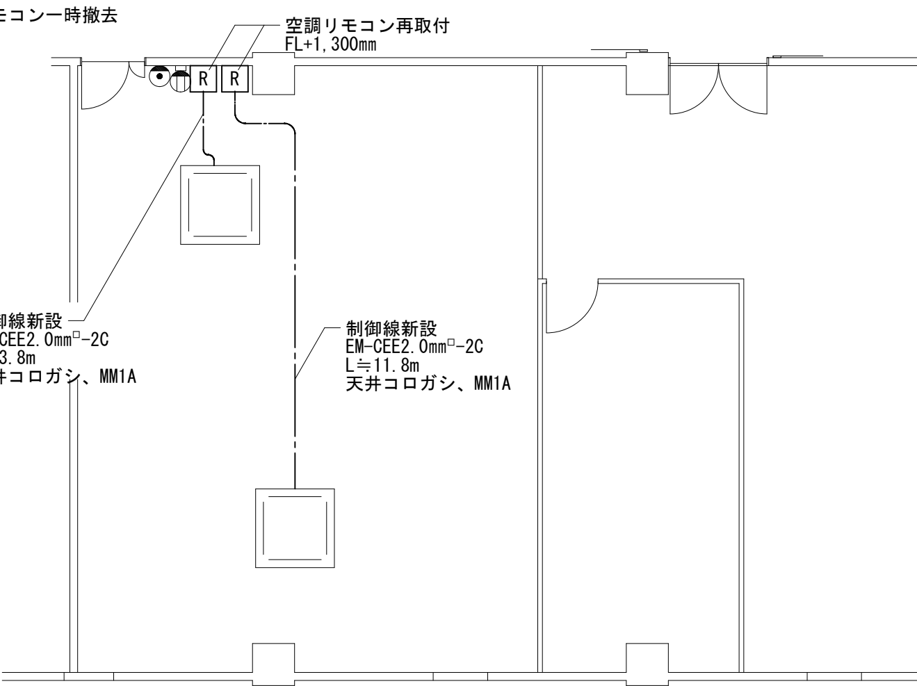
施工箇所⑦設備平面詳細図(改修後) S=1/100
