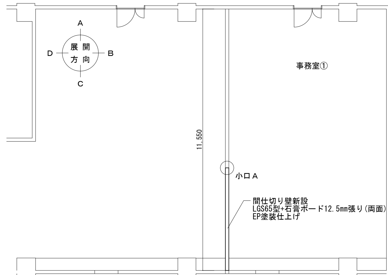
施工箇所①平面詳細図(改修後) S=1/100
