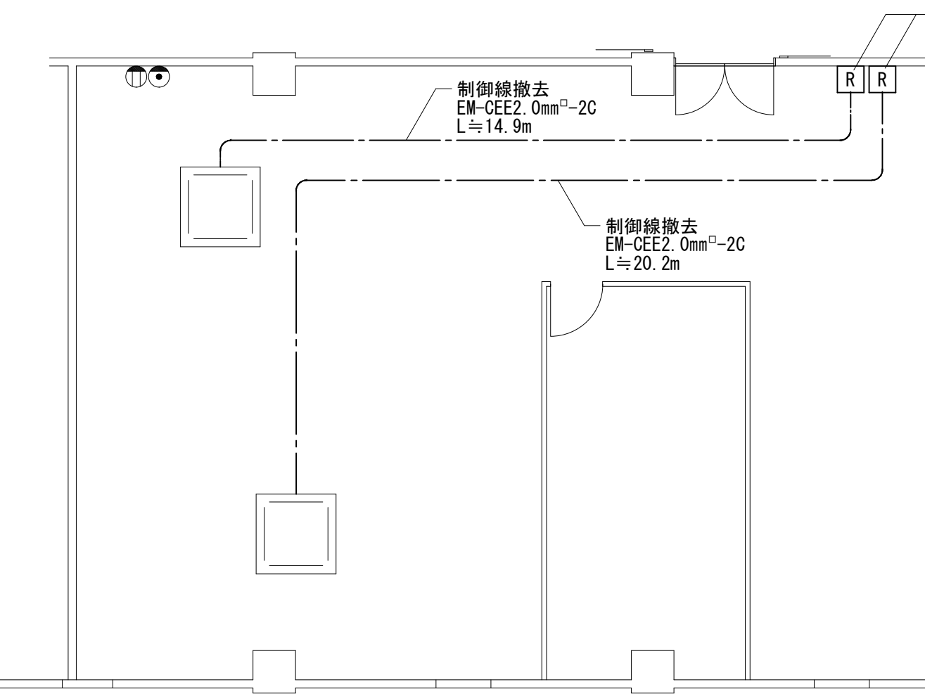
施工箇所⑦設備平面詳細図(改修前) S=1/100
