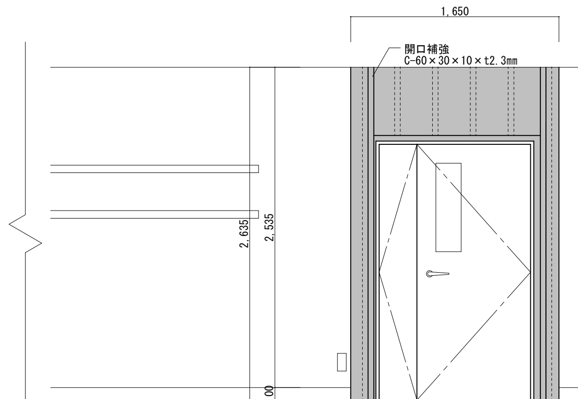
施工箇所②廊下展開図A(改修後) S=1/30
