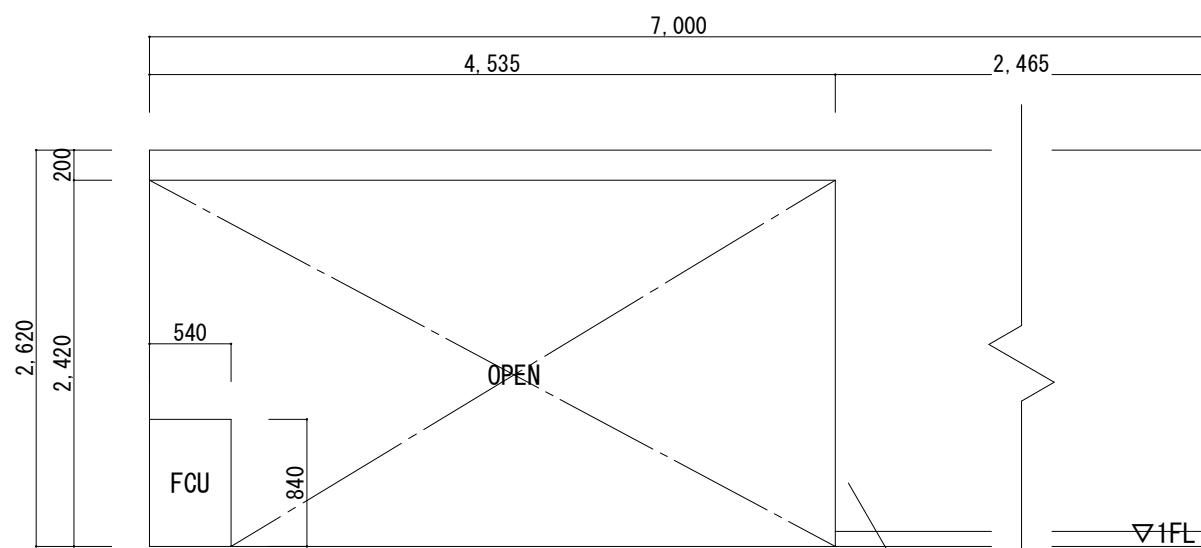
事務室①展開図D(改修前) S=1/50
