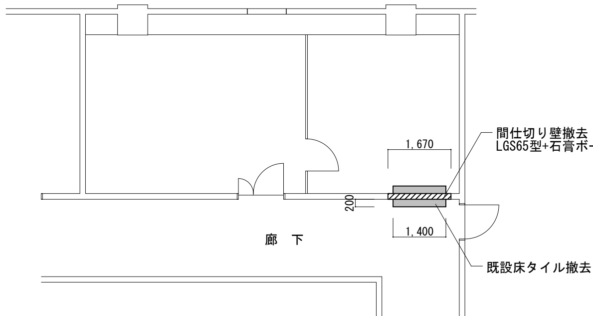
施工箇所②平面詳細図(改修前) S=1/100
