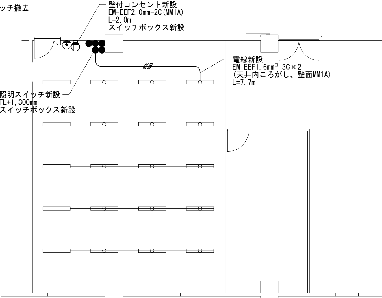
施工箇所⑦設備平面詳細図(改修後) S=1/100
