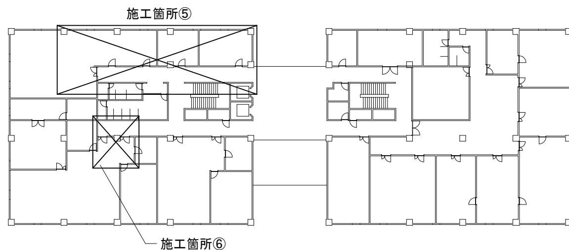
154号建物3階キープラン S=1/500
