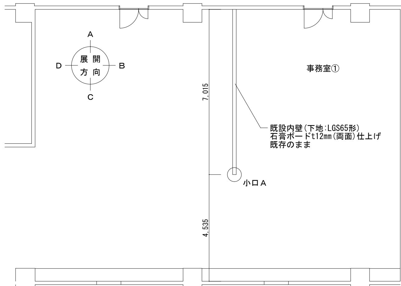
施工箇所①平面詳細図(改修前) S=1/100
