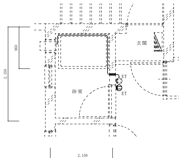
電気設備改修展開図 S=1/X
