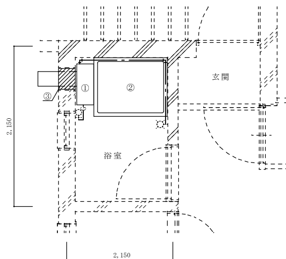
〔改修後〕施工箇所平面図 S=1/60
