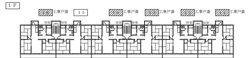
健軍宿舎8号棟平面図 S=1/400
