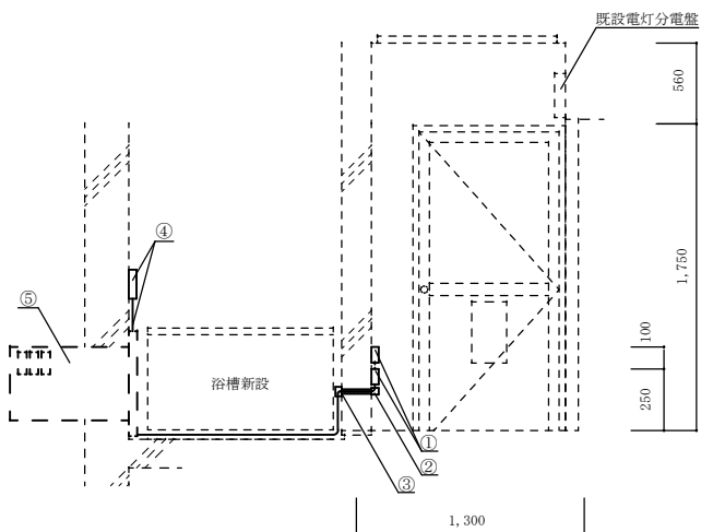
電気設備改修展開図 S=1/X
