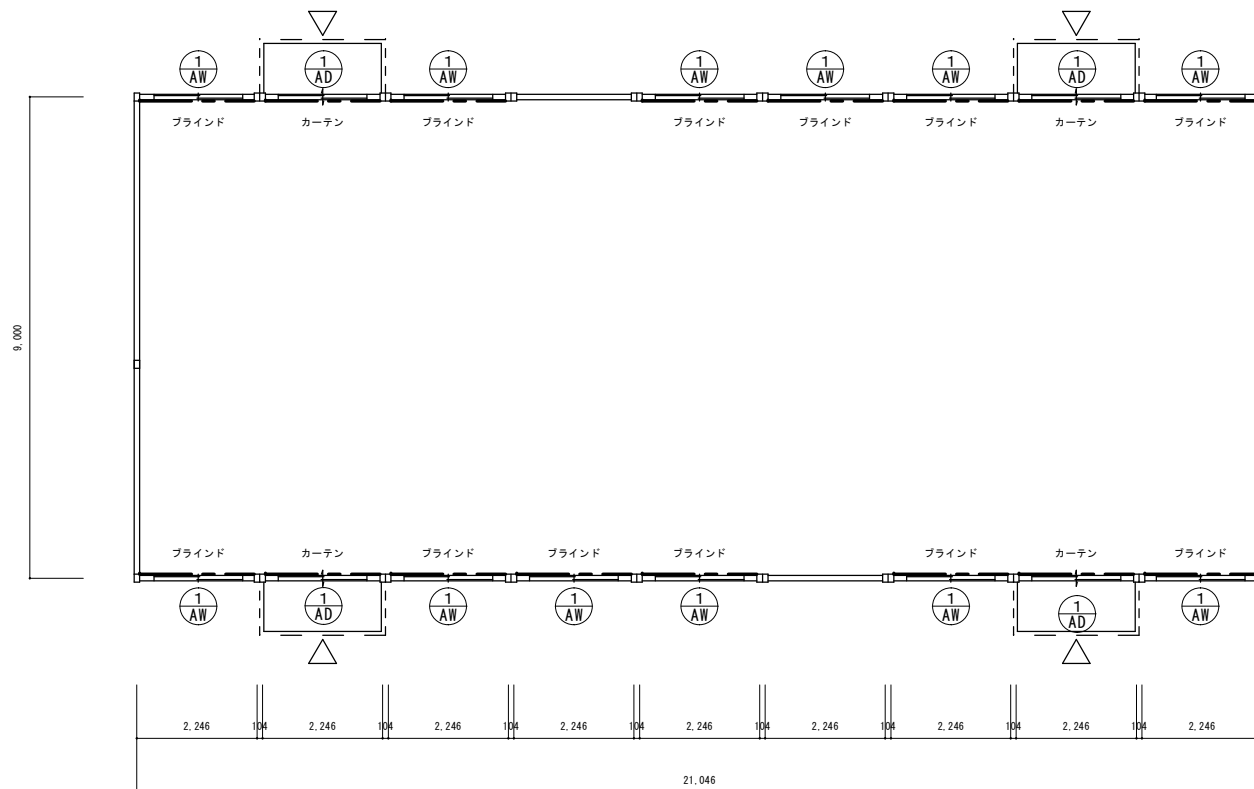
平面図 S=1:100
