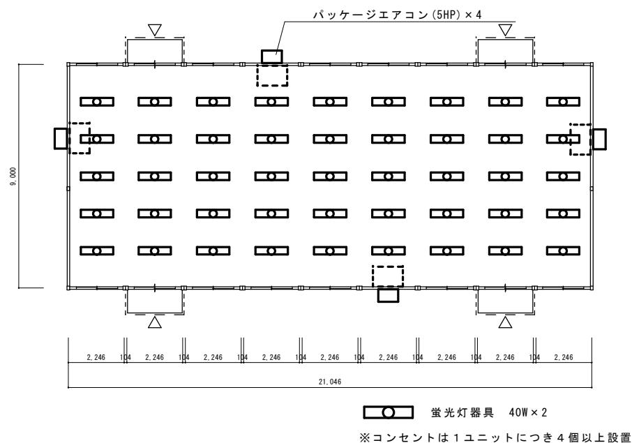
平面図 S=1:150
