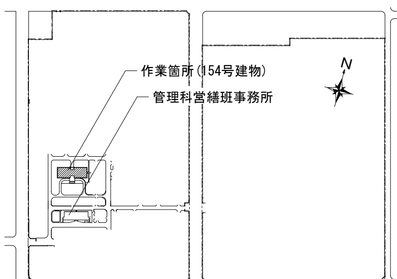
駐屯地配置図 S=1/10,000
