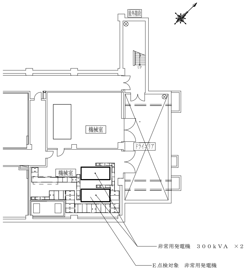
1号庁舎平面図 1/200
