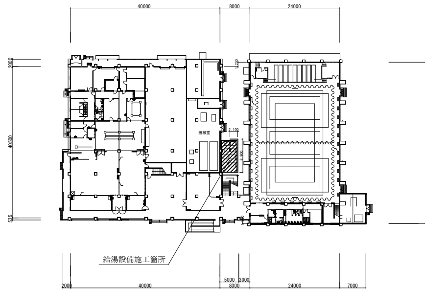
8号建物 1階平面図 S=1/800
