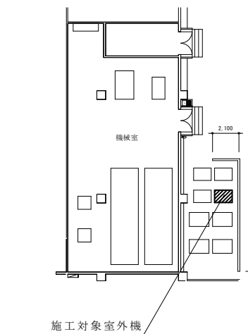
機械室外 平面図 S=1/300
