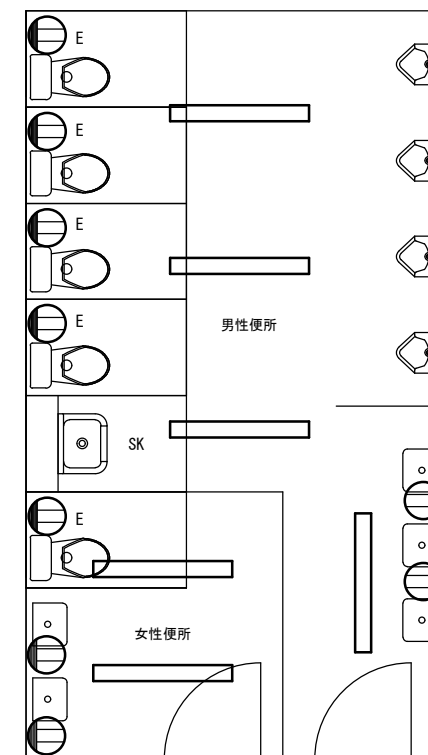
便所詳細図 S=1/50
