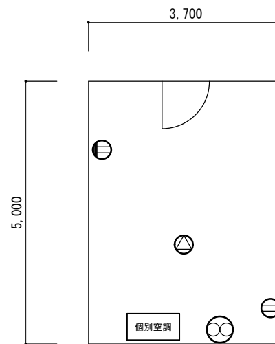
自習室標準図
