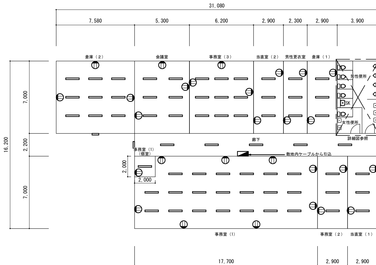
平面図 S=1/150
