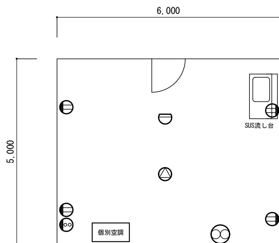
娯楽室標準図
