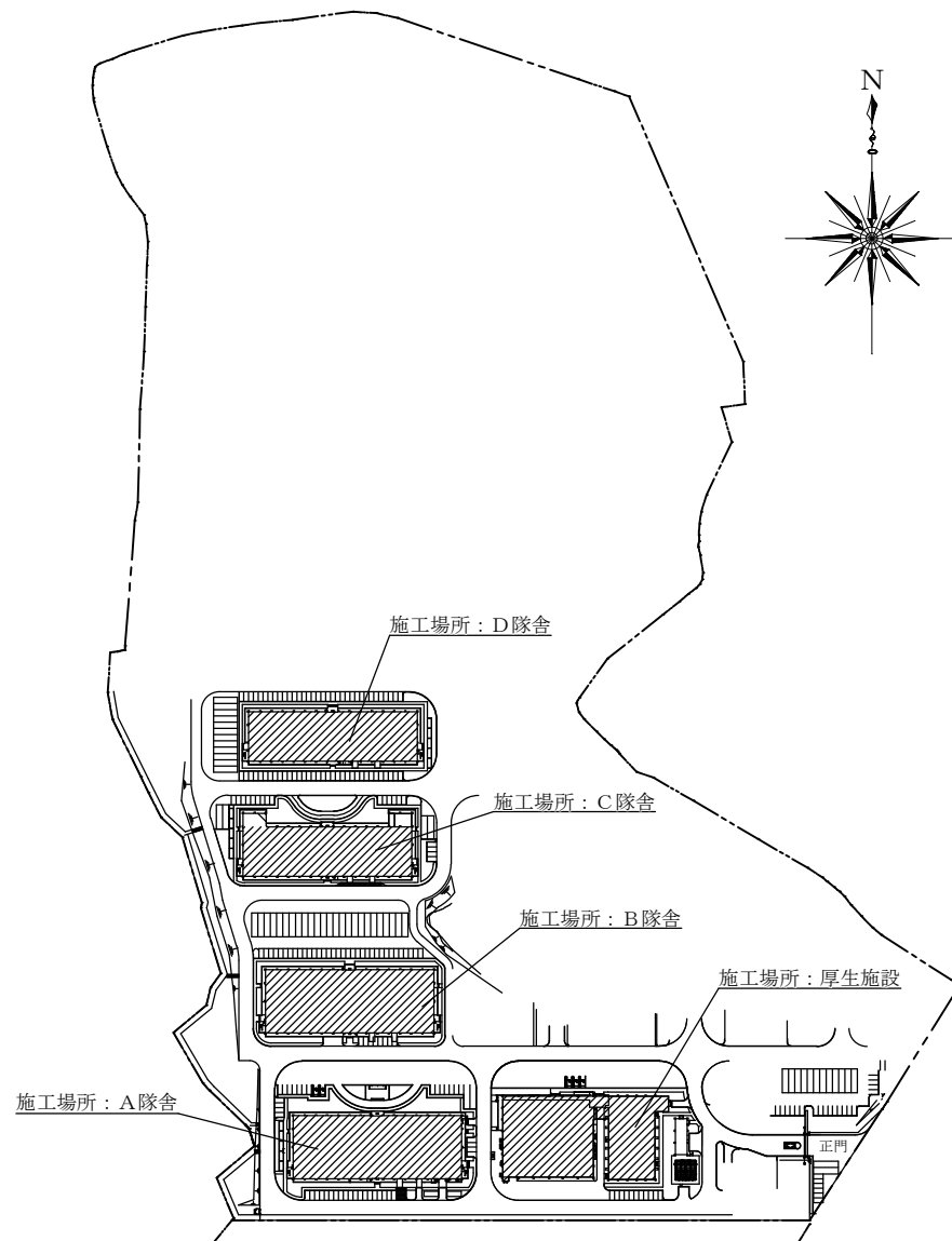
配置図 S=1/3,000
