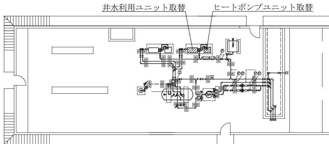
C・D隊舎屋上既設衛生設備平面図 1/150
