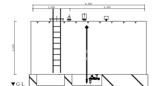
受水槽背面図 1/75
