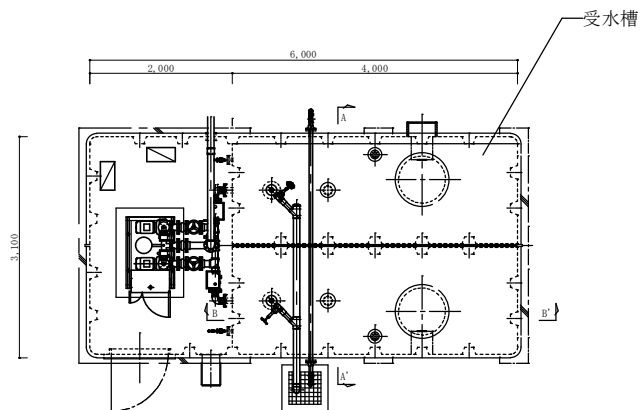
受水槽平面図 1/75
