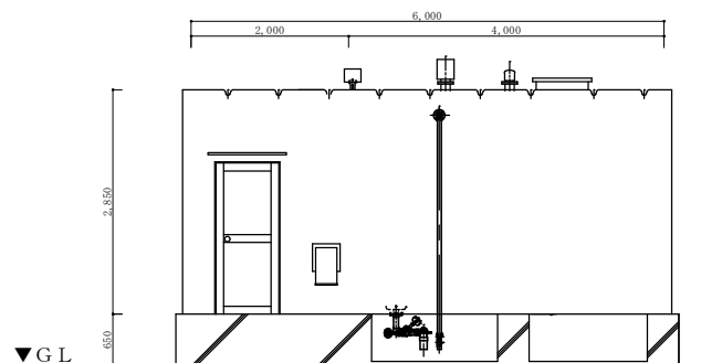
受水槽正面図 1/75
