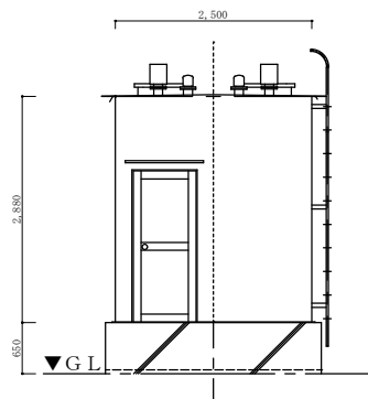
受水槽正面図 1 / 7 5
