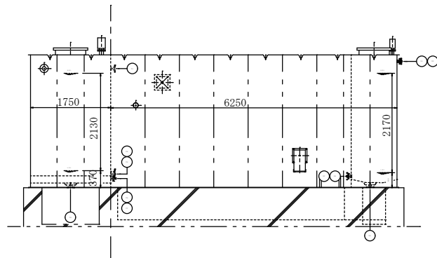
受水槽側面図 1 / 7 5
