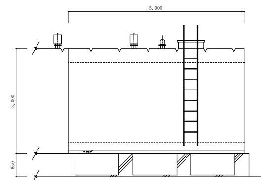
B-B'断面図 1 / 7 5
