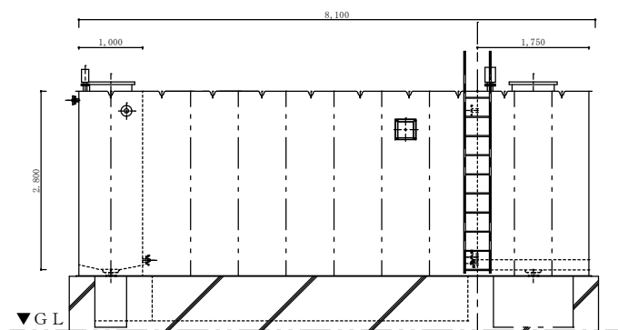
受水槽側面図 1 / 7 5
