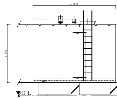
B-B'断面図 1/75
