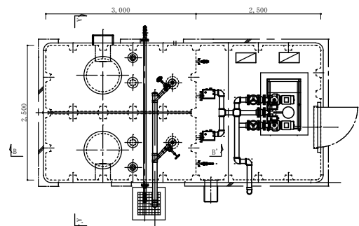
受水槽平面図 1 / 7 5
