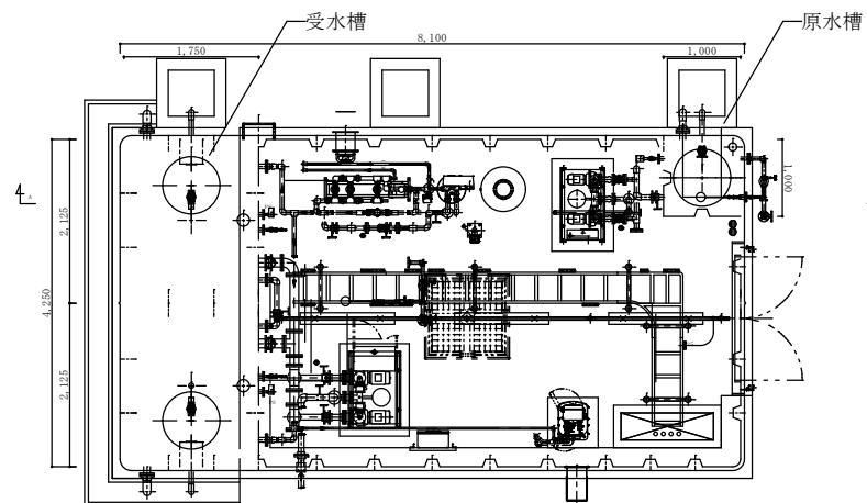
受水槽平面図 1 / 7 5
