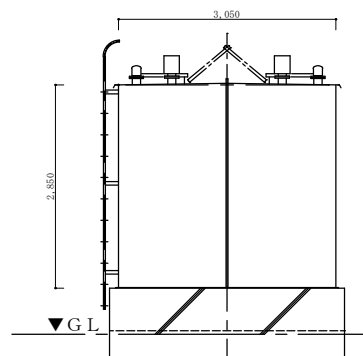
A-A'断面図 1/75
