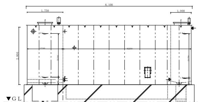
受水槽側面図 1 / 7 5
