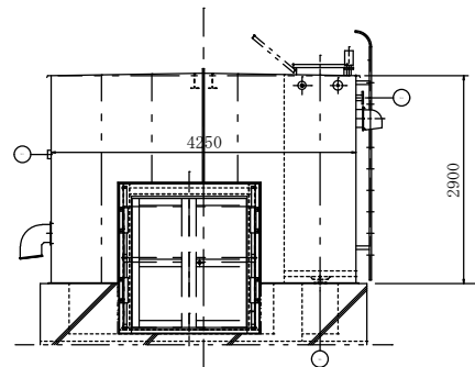
受水槽正面図 1 / 7 5
