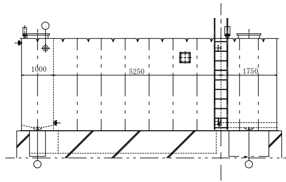
受水槽側面図 1 / 7 5
