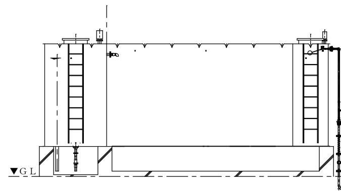
A-A断面図 1 / 7 5
