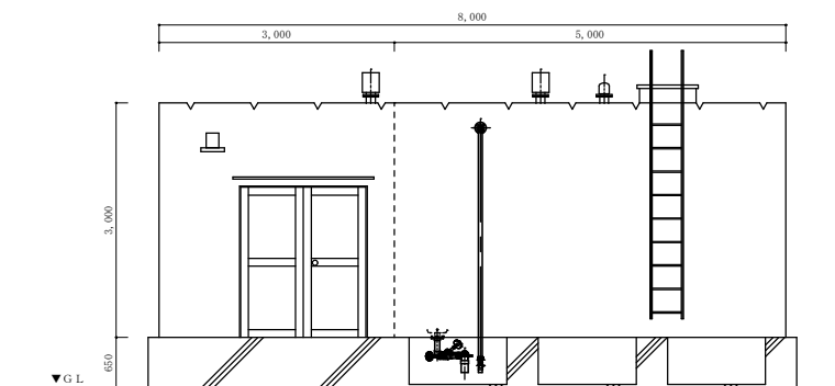
受水槽正面図 1 / 7 5
