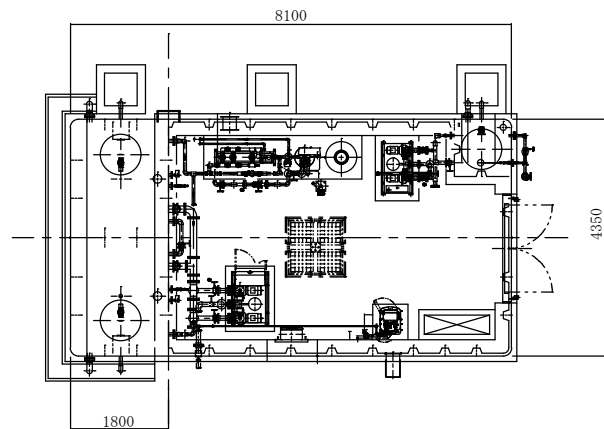
受水槽平面図 1 / 7 5
