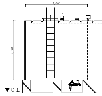
B-B'断面図 1 / 7 5
