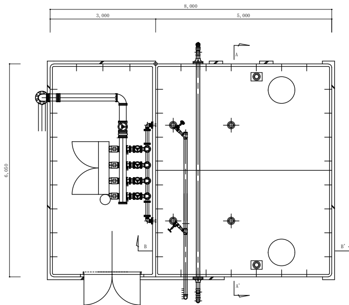
受水槽平面図 1 / 7 5
