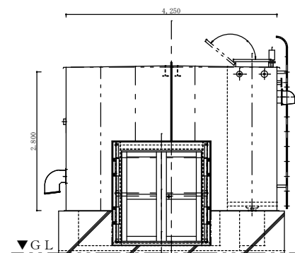
受水槽正面図 1 / 7 5
