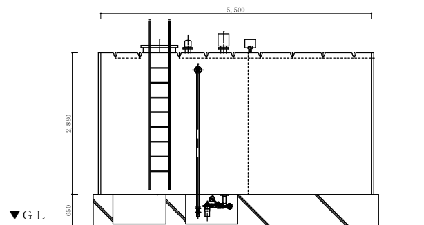
受水槽背面図 1 / 7 5
