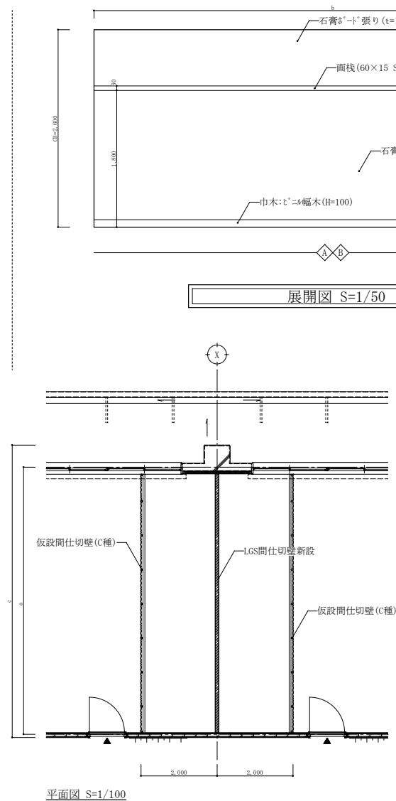
仮設計画図
