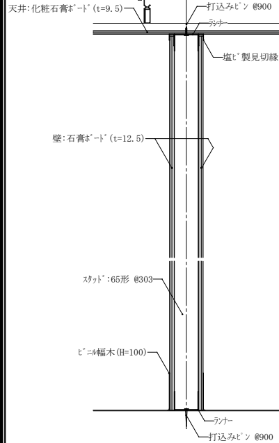
画栈詳細図
