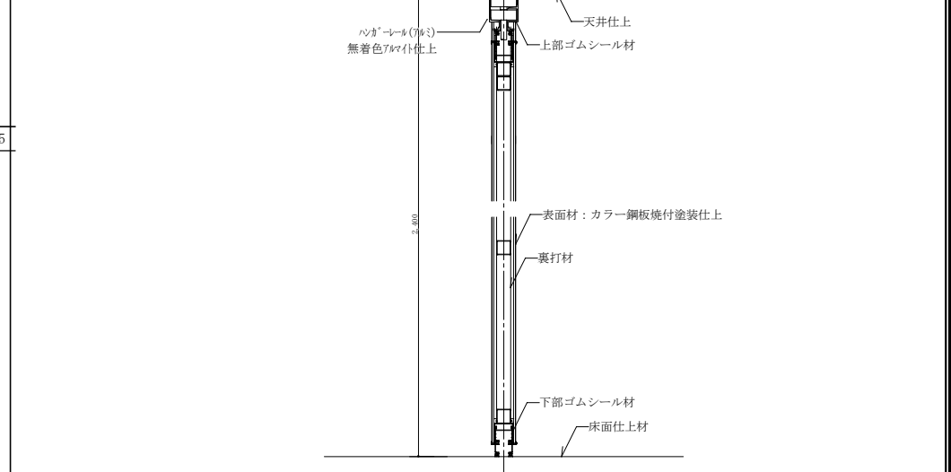
建具詳細図
