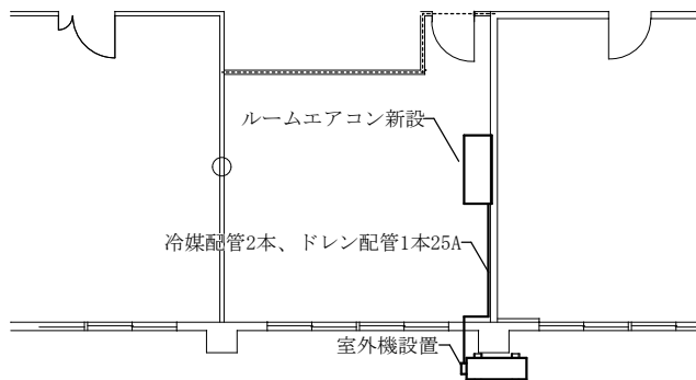
C庁舎2階平面図 S=1/75
