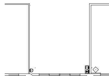
C庁舎2階通信配線既設平面図 S=1/150
