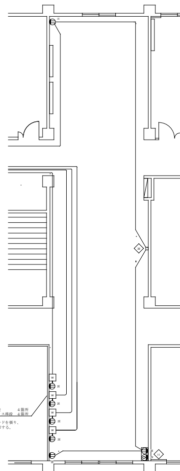
C庁舎2階電気設備撤去平面図 S=1/150
