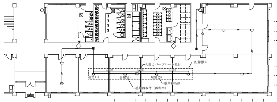
隊庁舎D1F 消防設備改修平面図 1/300
