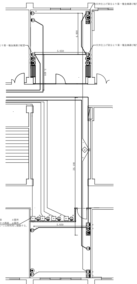
C庁舎2階電気設備改修平面図 S=1/150
