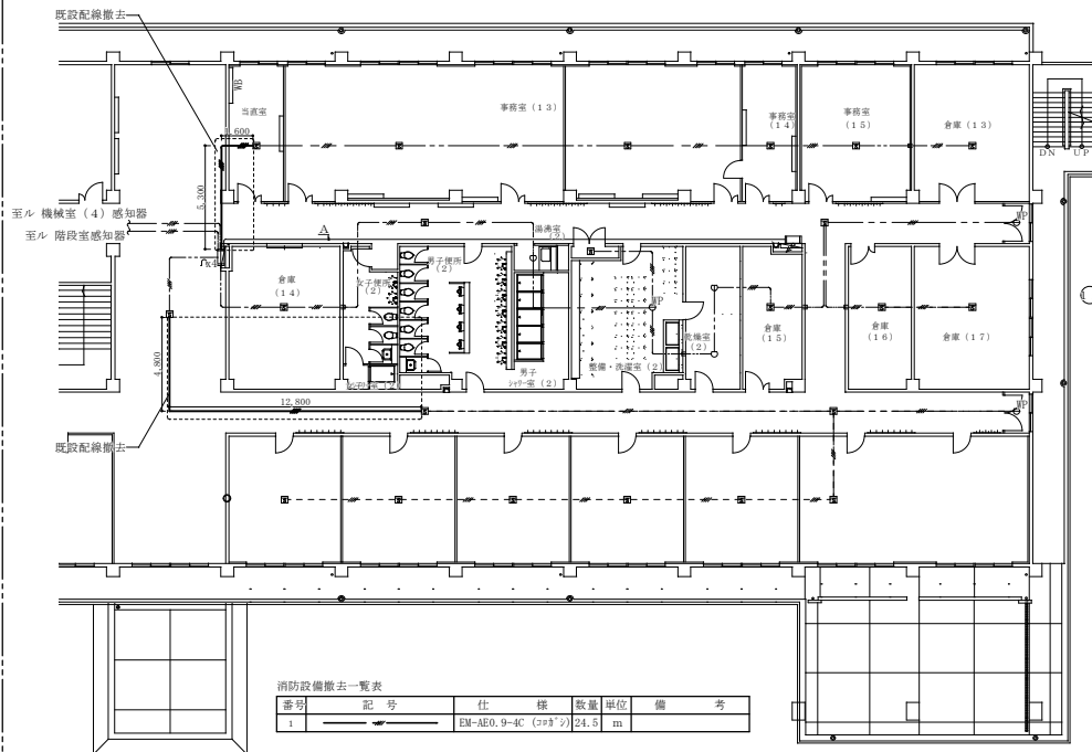
C庁舎2階消防設備撤去平面図 S=1/150
