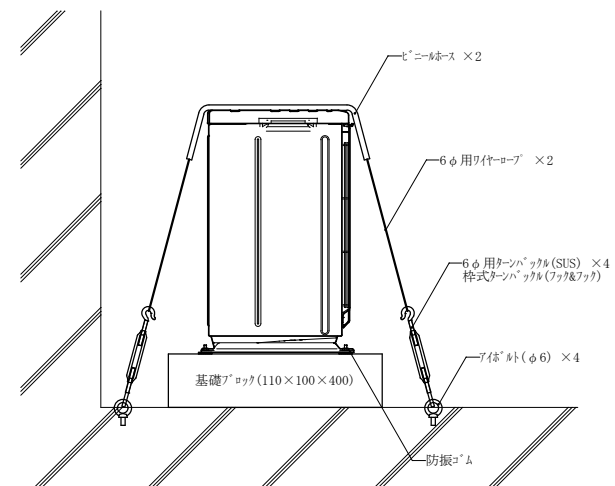
室外機基礎詳細図 S=1/10
