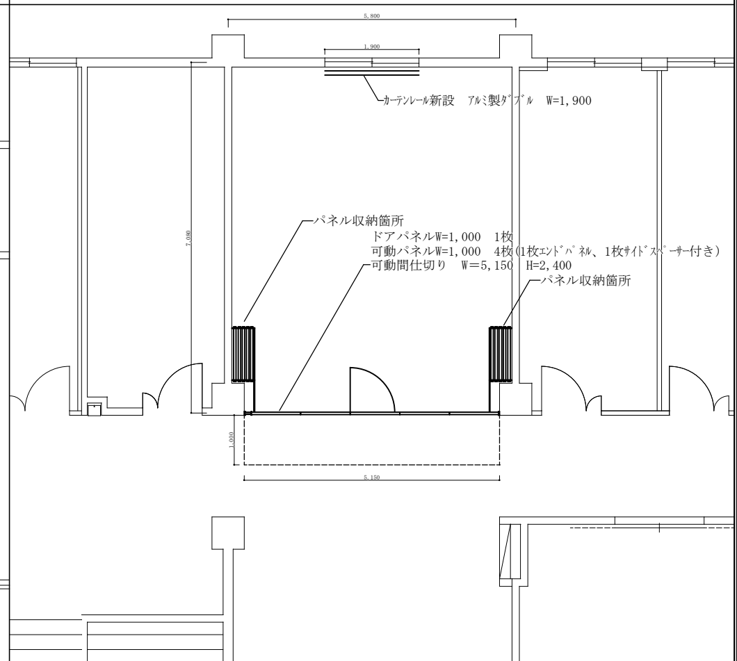
C庁舎2階平面図 S=1/75
