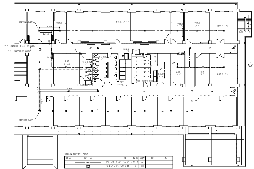
C庁舎2階消防設備改修平面図 S=1/150
