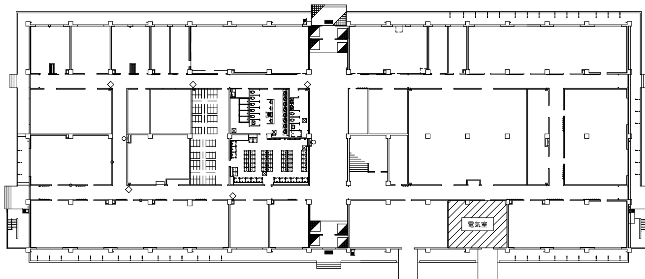
2号建物 1階平面図 NON SCALE
