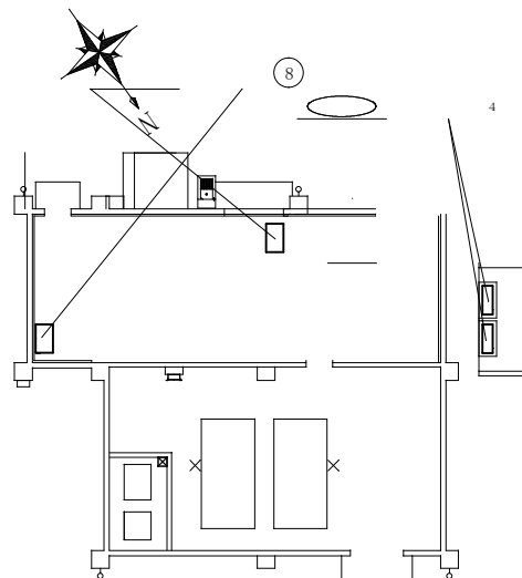
空調設備平面図 (3号) 1/200
