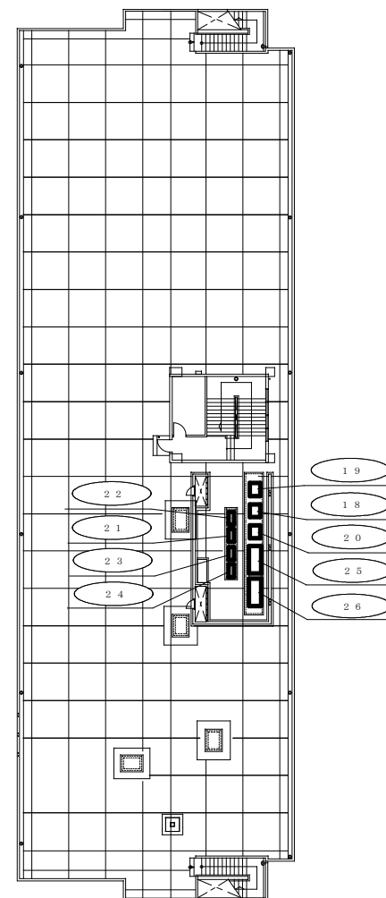
空調設備平面図 (15号RF) 1/350
