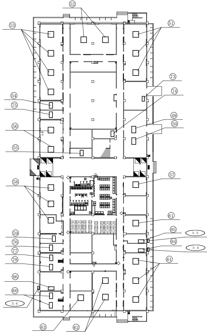
空調設備平面図 (2号1F) 1/500
