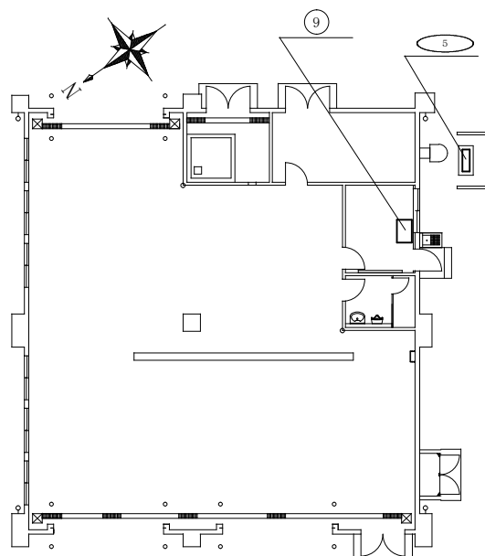
空調設備平面図 (4号) 1/200
