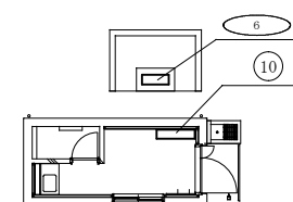
空調設備平面図 (6号) 1/150
