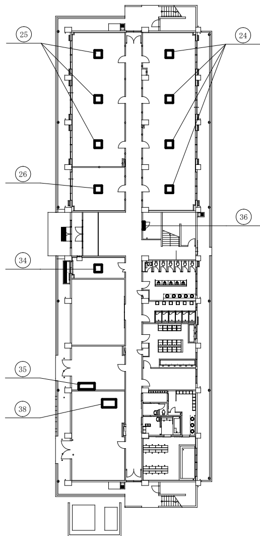
空調設備平面図 (15号1F) 1/350
