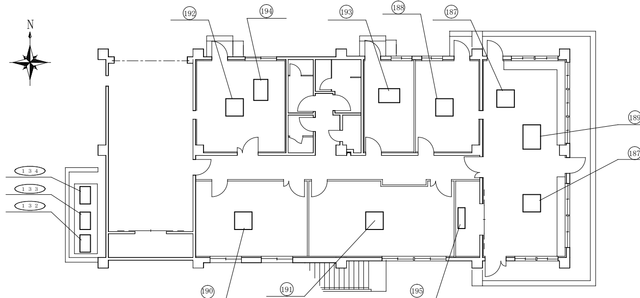
空調設備平面図 (7号) 1/150
