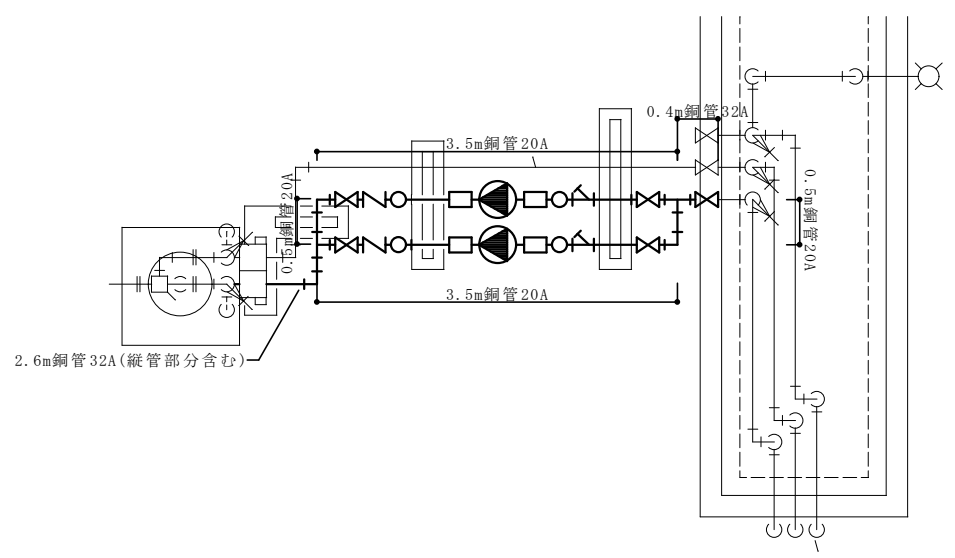
屋上配管詳細図 1 / 50
