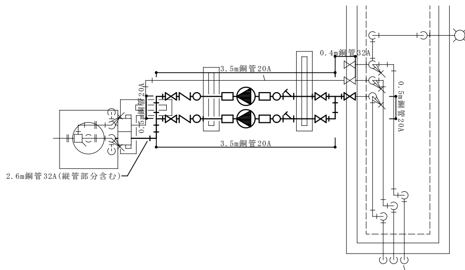
屋上配管詳細図 1 / 50
