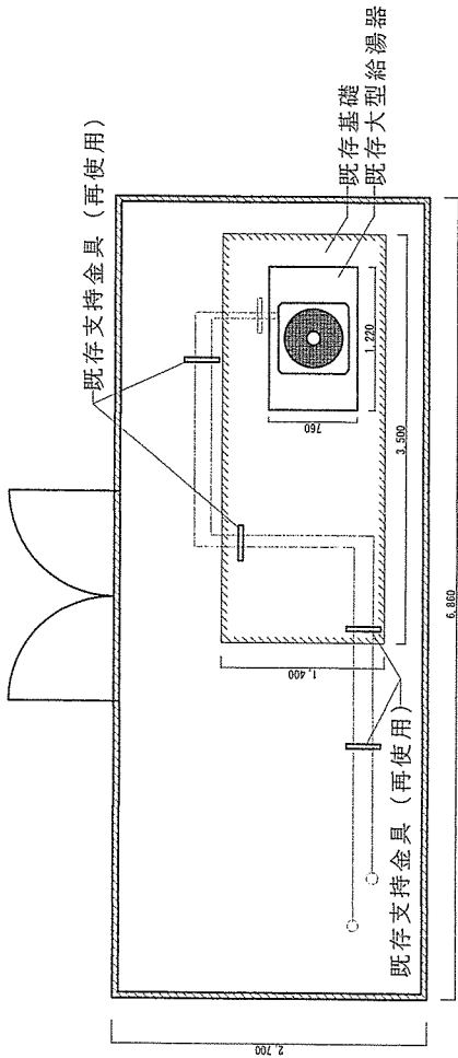
既存大型給湯器設置平面図 (S=1/50)
