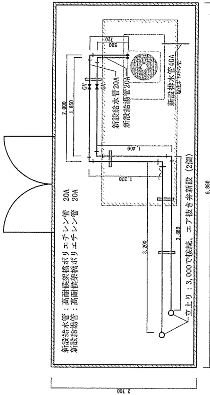
新設配管平面図 (S=1/50)
