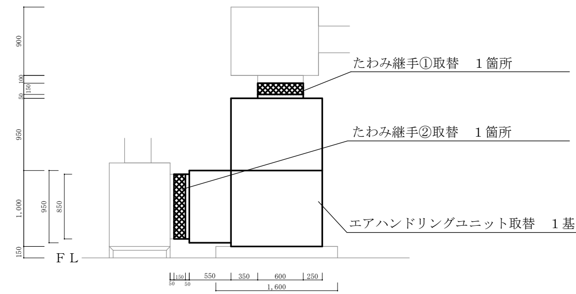
立面図【A面】 S=1/50
