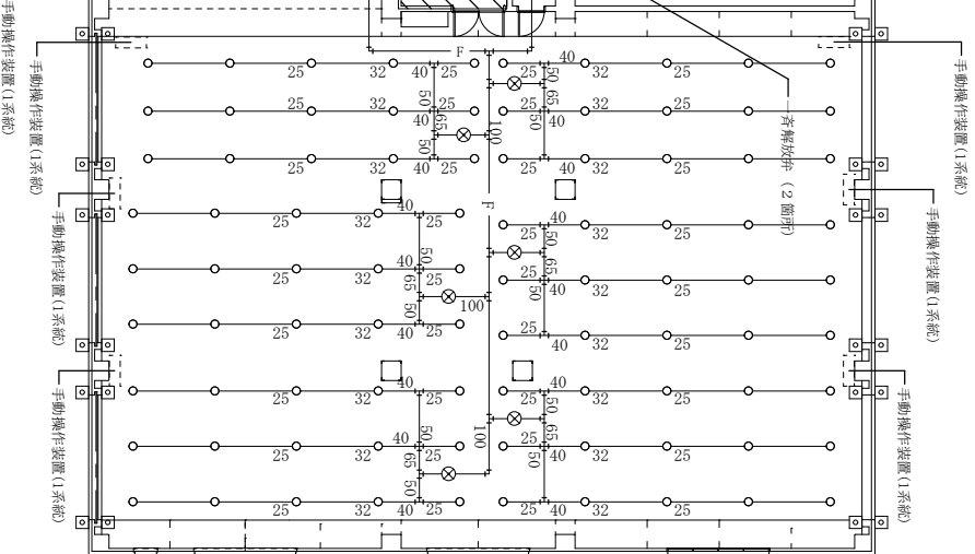
建第22号建物平面図 S=1/300
