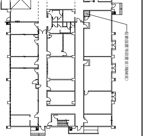
平面図 S=1/500
