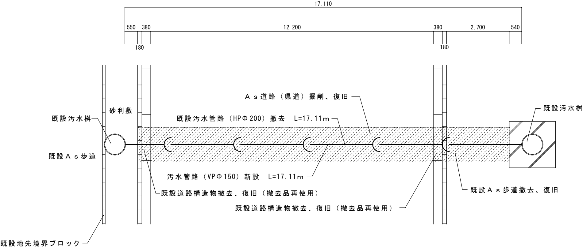
汚水管路配置図 S=1/100
