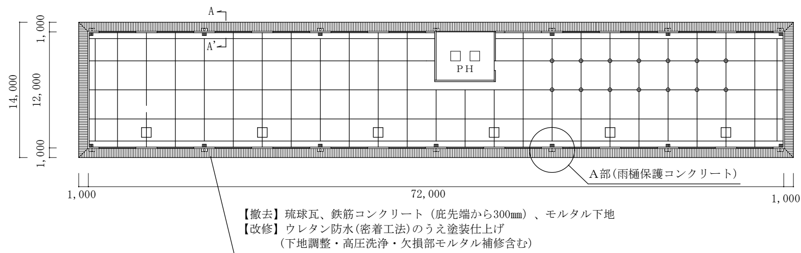
P H 屋根伏図 S=1/200
