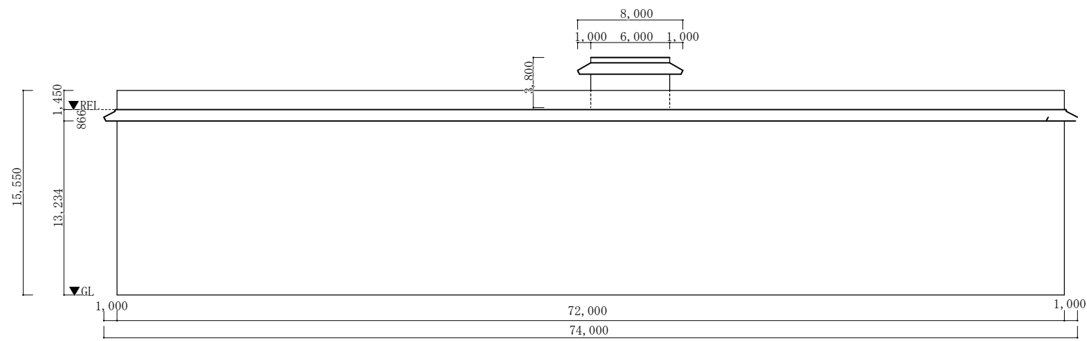
1 0 3 号隊舎立面図 S=1/400
