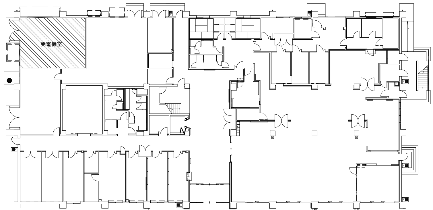
23号建物平面図 S=1:100
