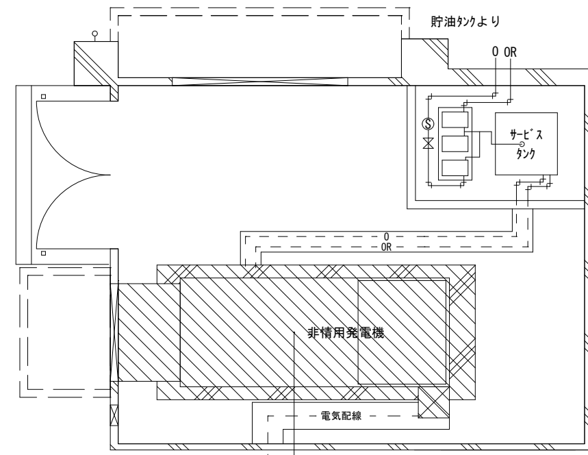
23号建物発電機室 S=1:100
