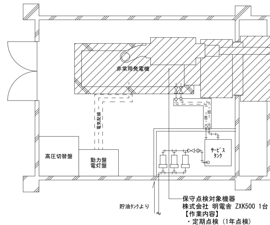
(白川) 平面図 S=1:100
