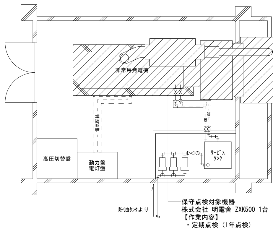
(八重瀬) 平面図 S=1:100
