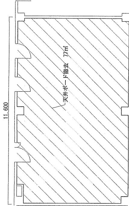
【施工前(天井)】2F平面詳細図 S=1/100
