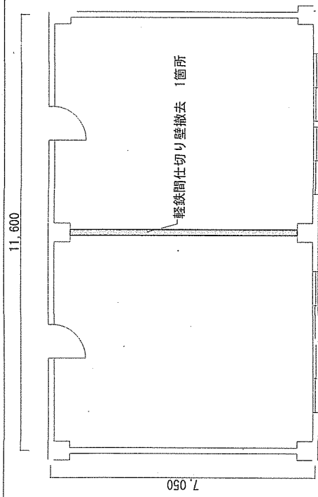
【施工前(間仕切)】3F平面詳細図 S=1/100
