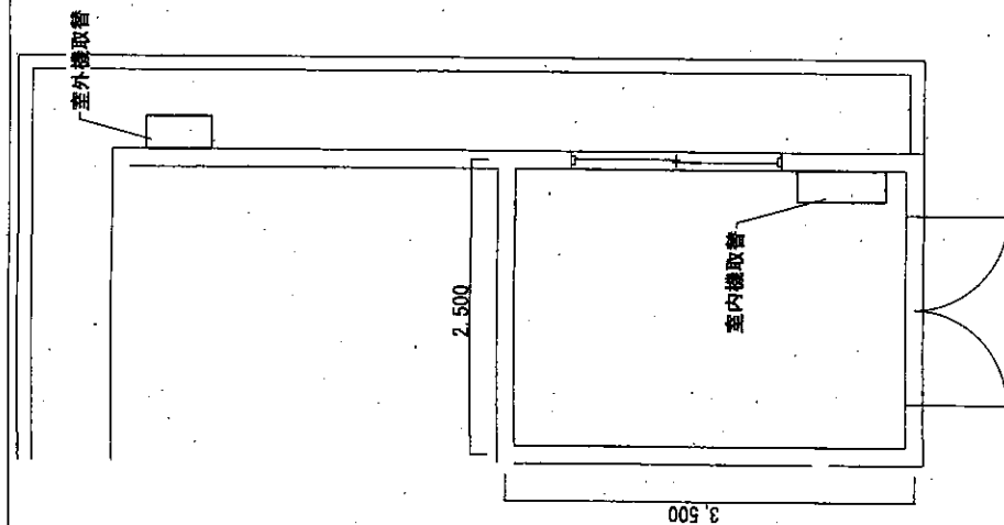
【施工場所①】平面詳細図 S=1/50
