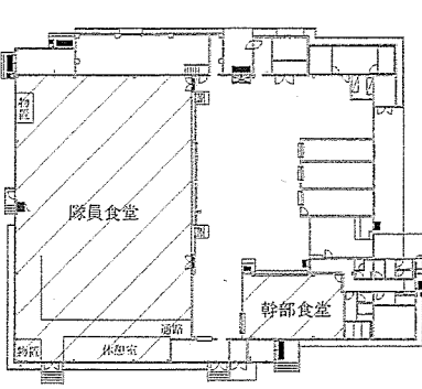
食堂平面図 1/700
