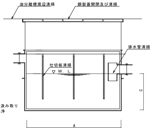
X-X' 断面図 S=Free
