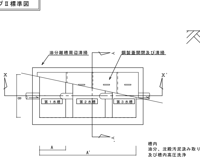
平面図 S=Free
