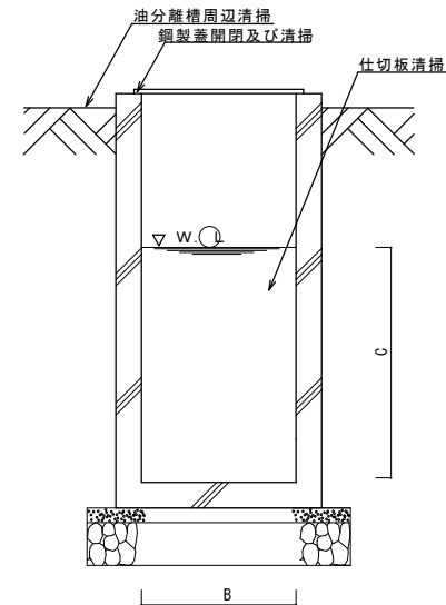
Y-Y' 断面図 S=Free
