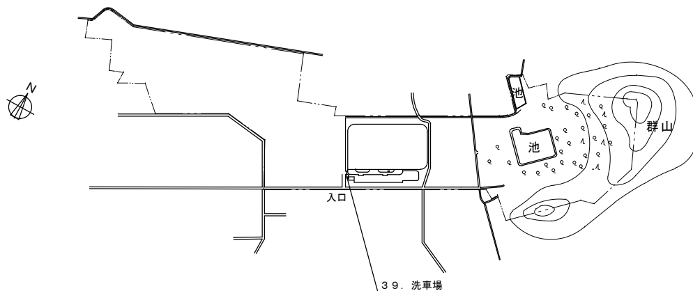
黒石原演習場油分離槽配置図 S=Free
