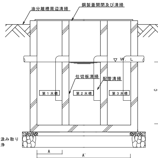
X-X' 断面図 S=Free
