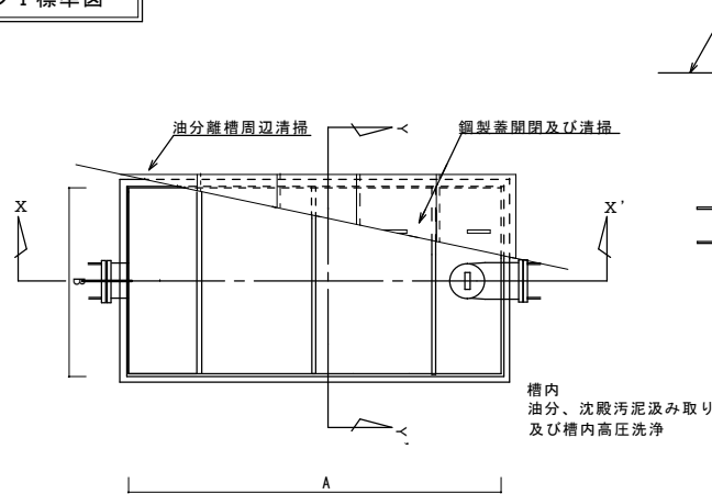
平面図 S=Free
