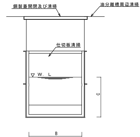
Y-Y' 断面図 S=Free
