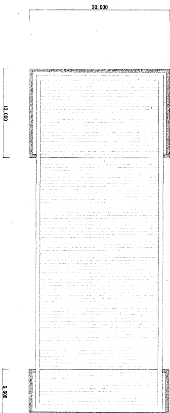
屋根伏図 S=1/500
