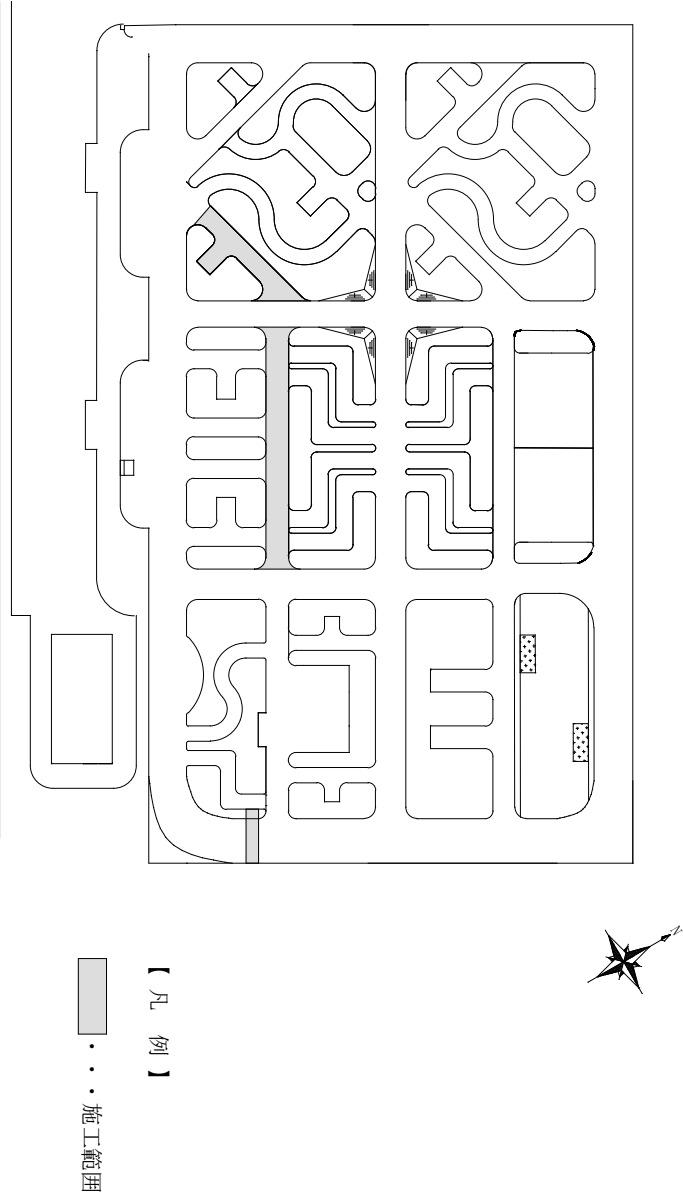
自動車訓練場配置図 S=1/2,000
