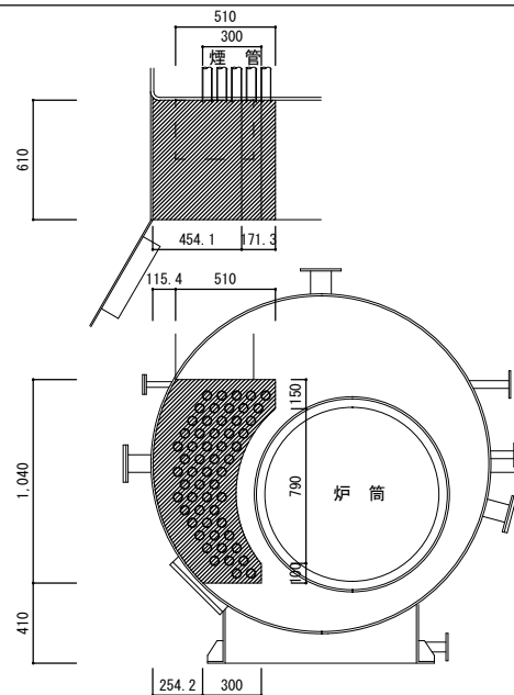
前煙室詳細図 S=1/30
