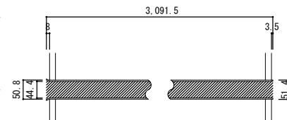
煙管詳細図 S=1/10
