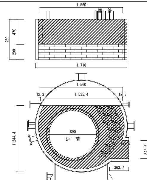
後煙室詳細図 S=1/30
