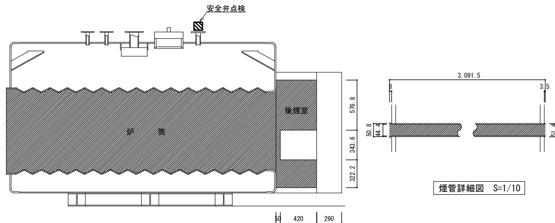
B～B' 断面図 S=1/30
