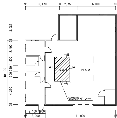
ボイラー室平面図 S=1/200
