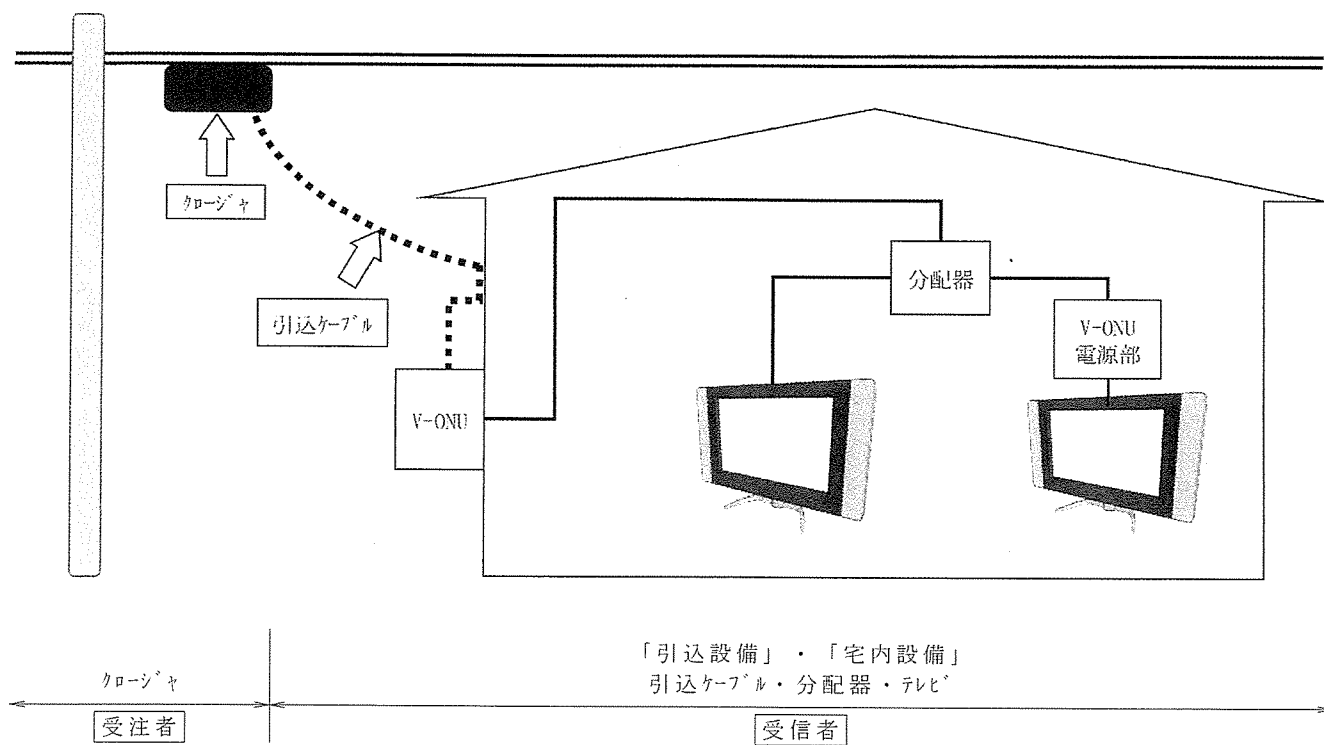
CATV設備保守管理範囲図
