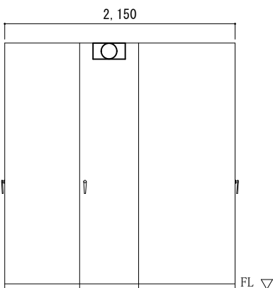
144号電気室CUB（左側面） 1：50
