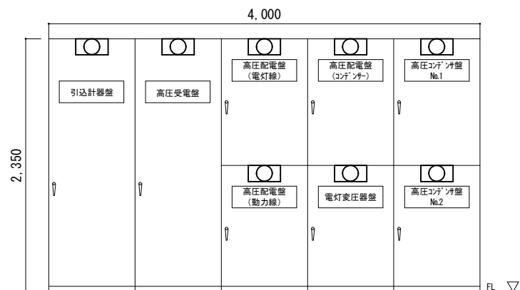
受電所CUB（正面） 1：50
