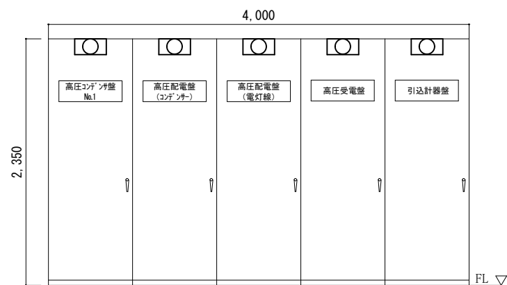
受電所CUB（裏面） 1：50
