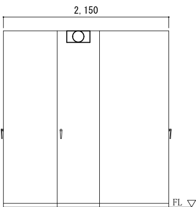
整備工場電気室CUB（右側面） 1：50
