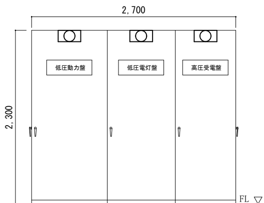
144号電気室CUB（裏面） 1：50
