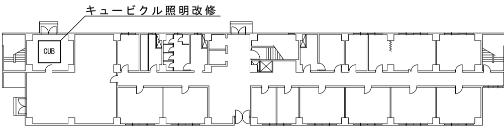
平面図
