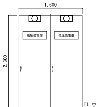
143号電気室CUB（裏面） 1：50
