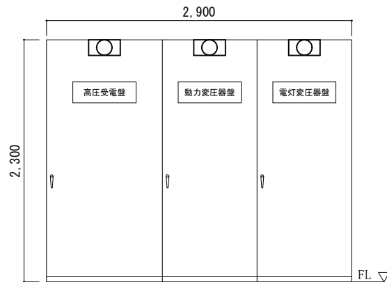
139号電氣室CUB（裏面） 1：50
