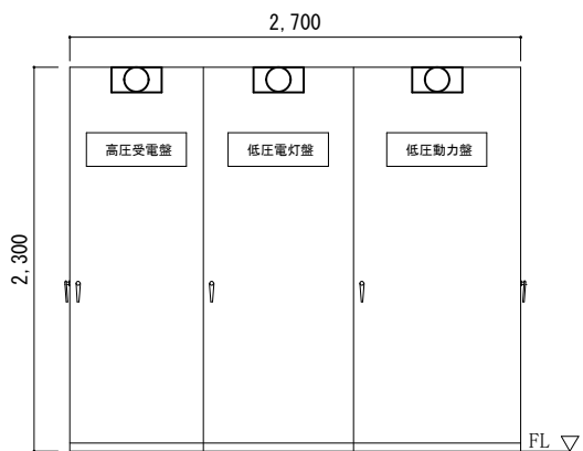
整備工場電気室CUB（正面） 1：50
