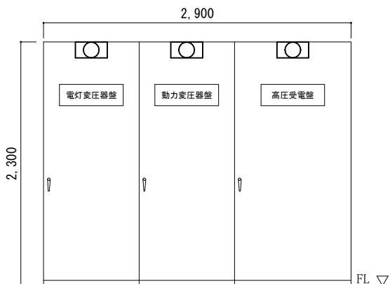
139号電氣室CUB（正面） 1：50
