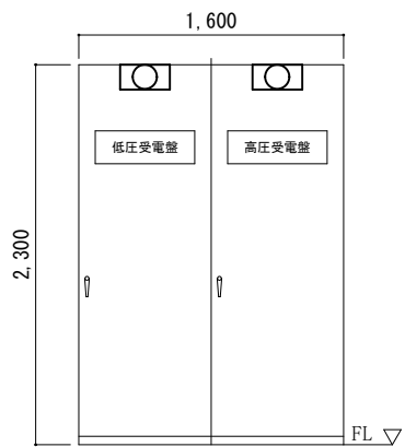
143号電気室CUB（正面） 1：50
