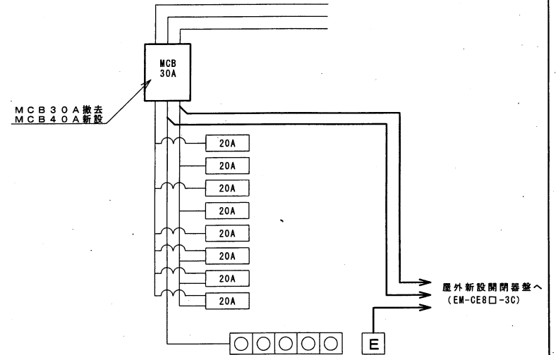
既設分電盤結線配線図 S=1/X
