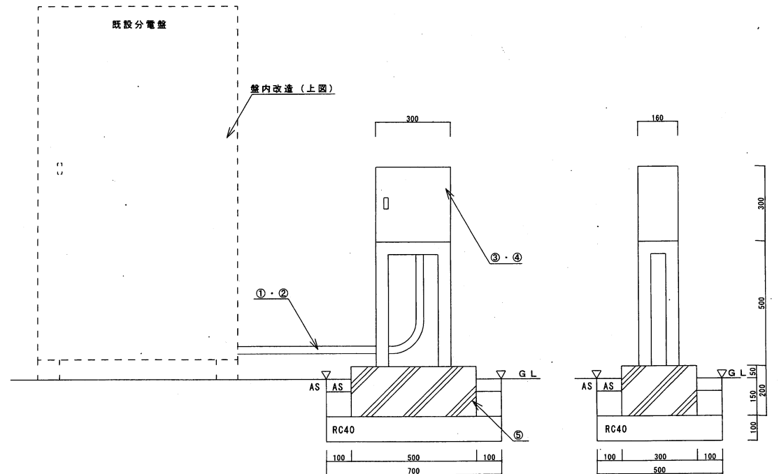
分電盤・開閉器盤立面図 S=1/15
