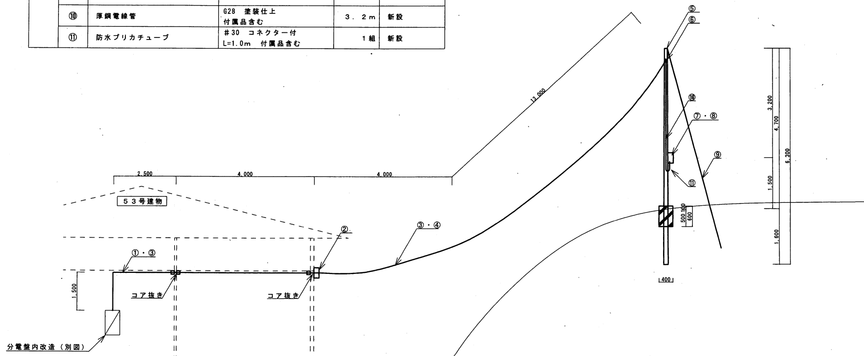
C地区 立面図 S=1/X
