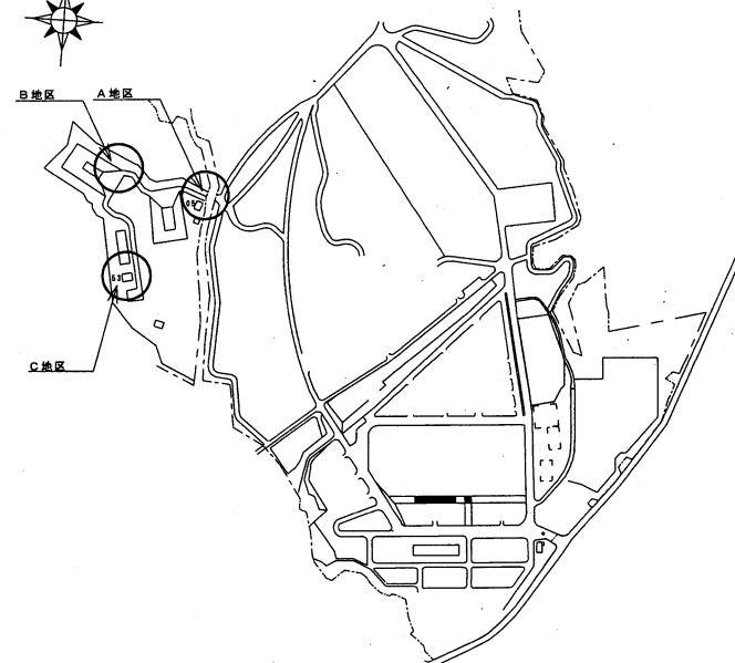
配置図 S=1/X
