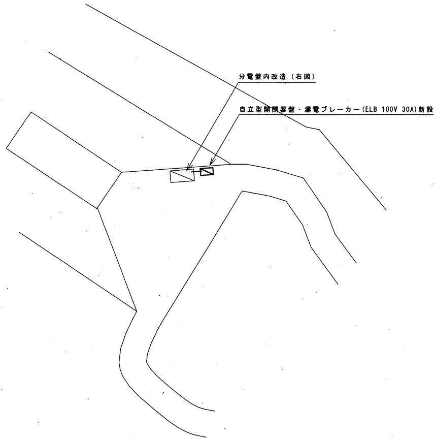
B 地区 配置図 S=1/30
