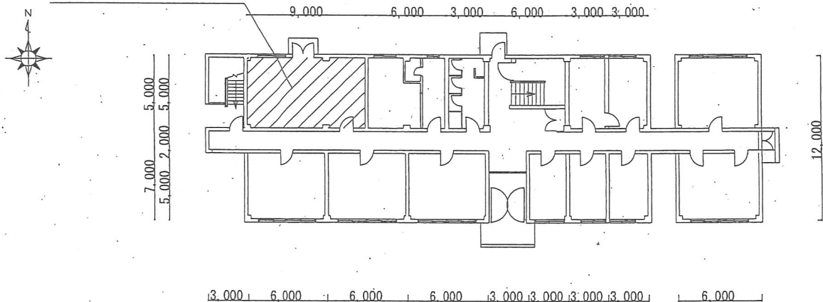
108号建物平面図 S=1/400
