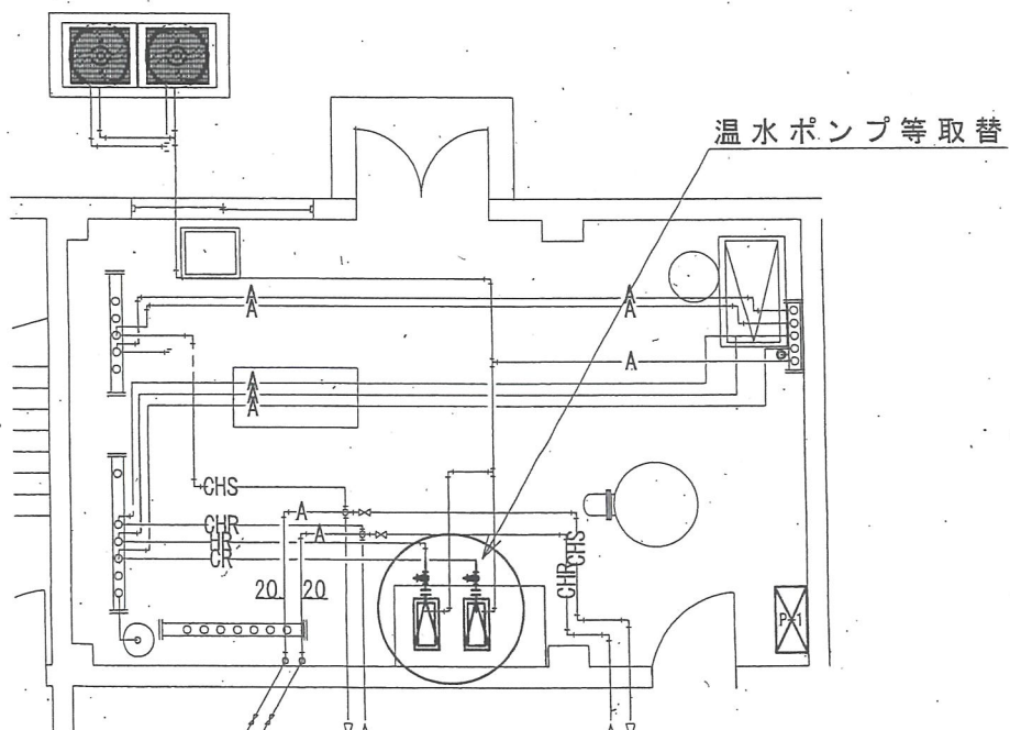
機械室平面図 S=1/100
