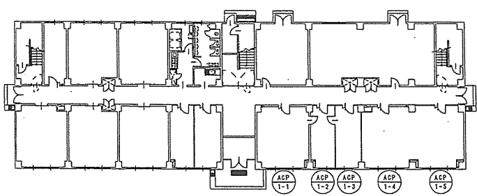
127号 建物平面図 S=1/600
