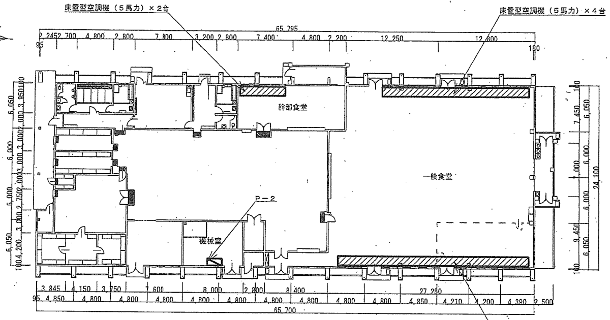
5号建物平面図 S=1/500
