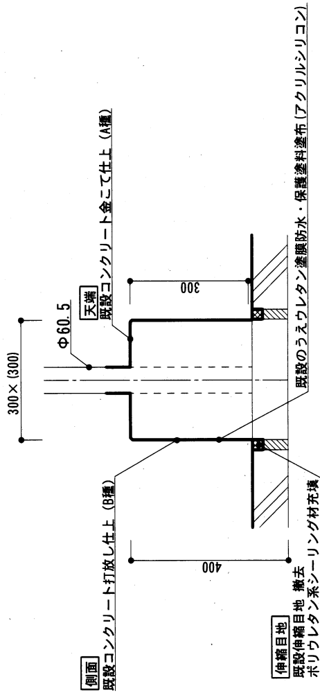
物干基礎断面詳細図
