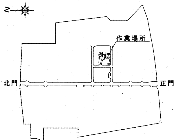
配置図 S=1/10000
