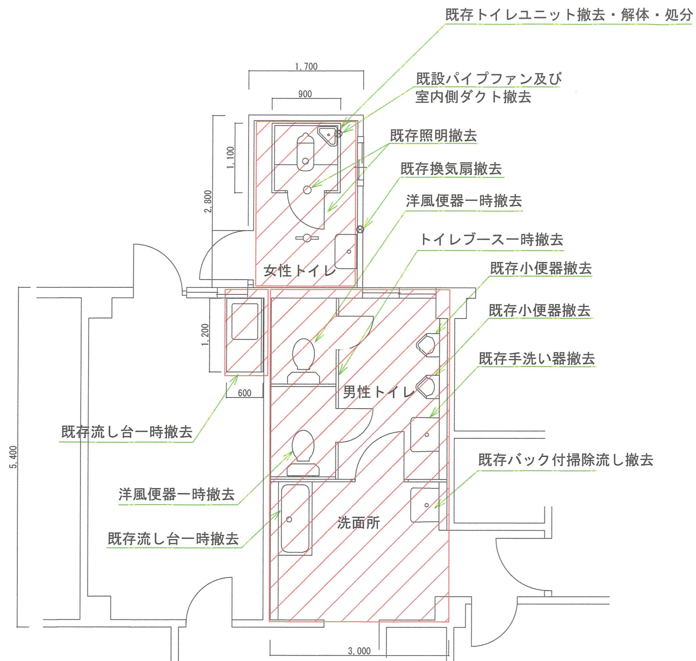
改修前平面図 S=1/60
