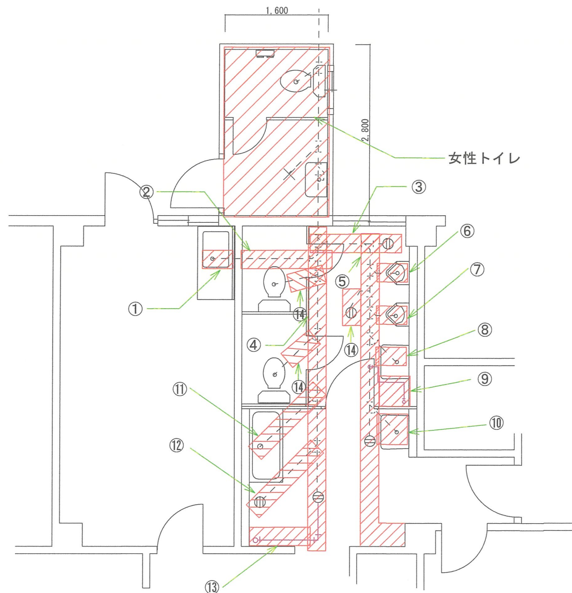
タイル補修等範囲平面図 S=1/60
