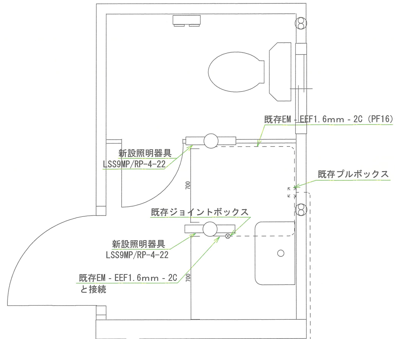
改修後平面図 S=1/20
