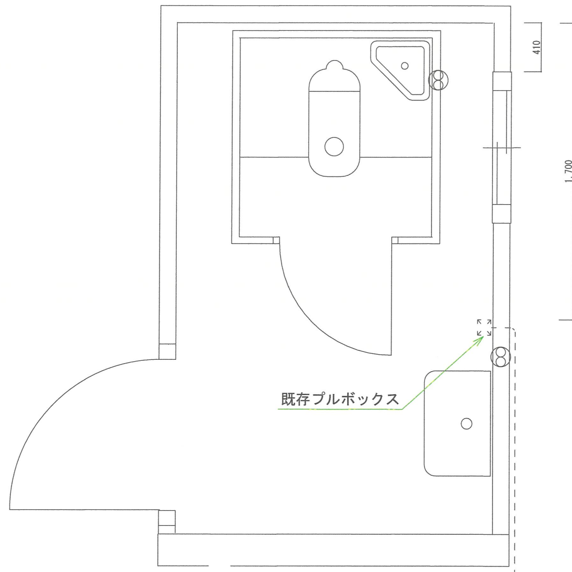
改修前平面図 S=1/20
