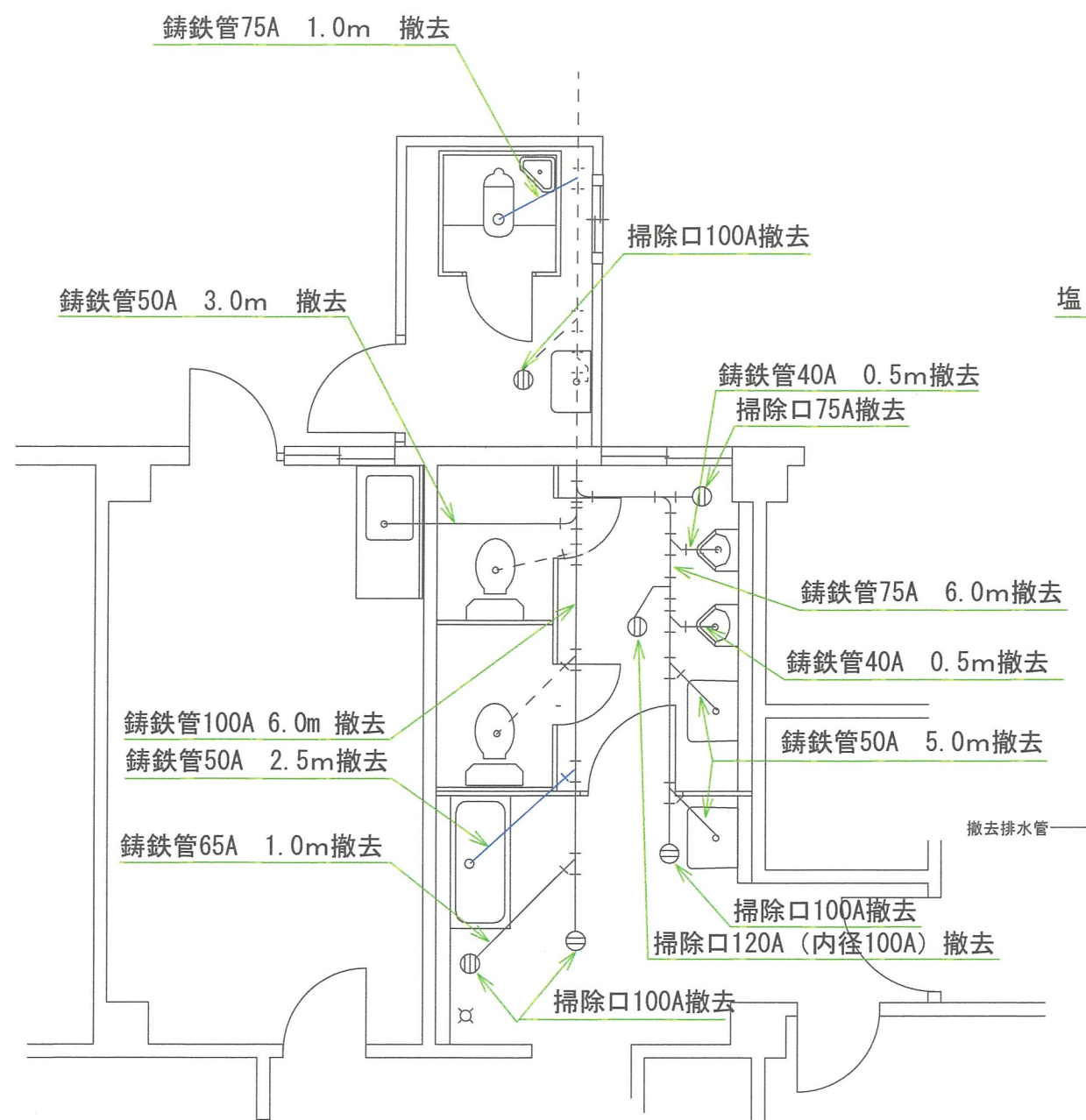
改修前平面図 S=1/60
