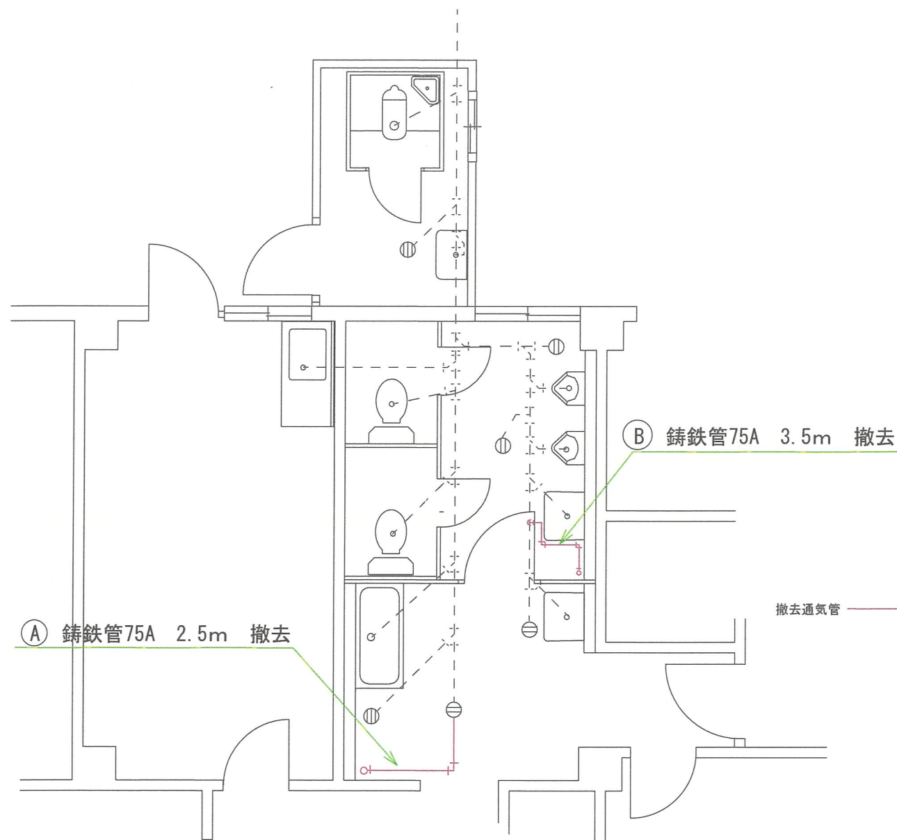
改修前平面図 S=1/60
