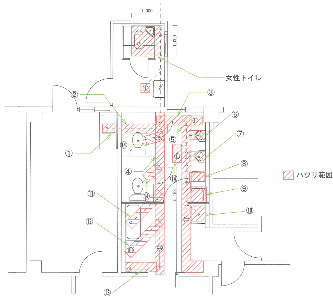
土間コンクリートハツリ範囲平面図 S=1/60
