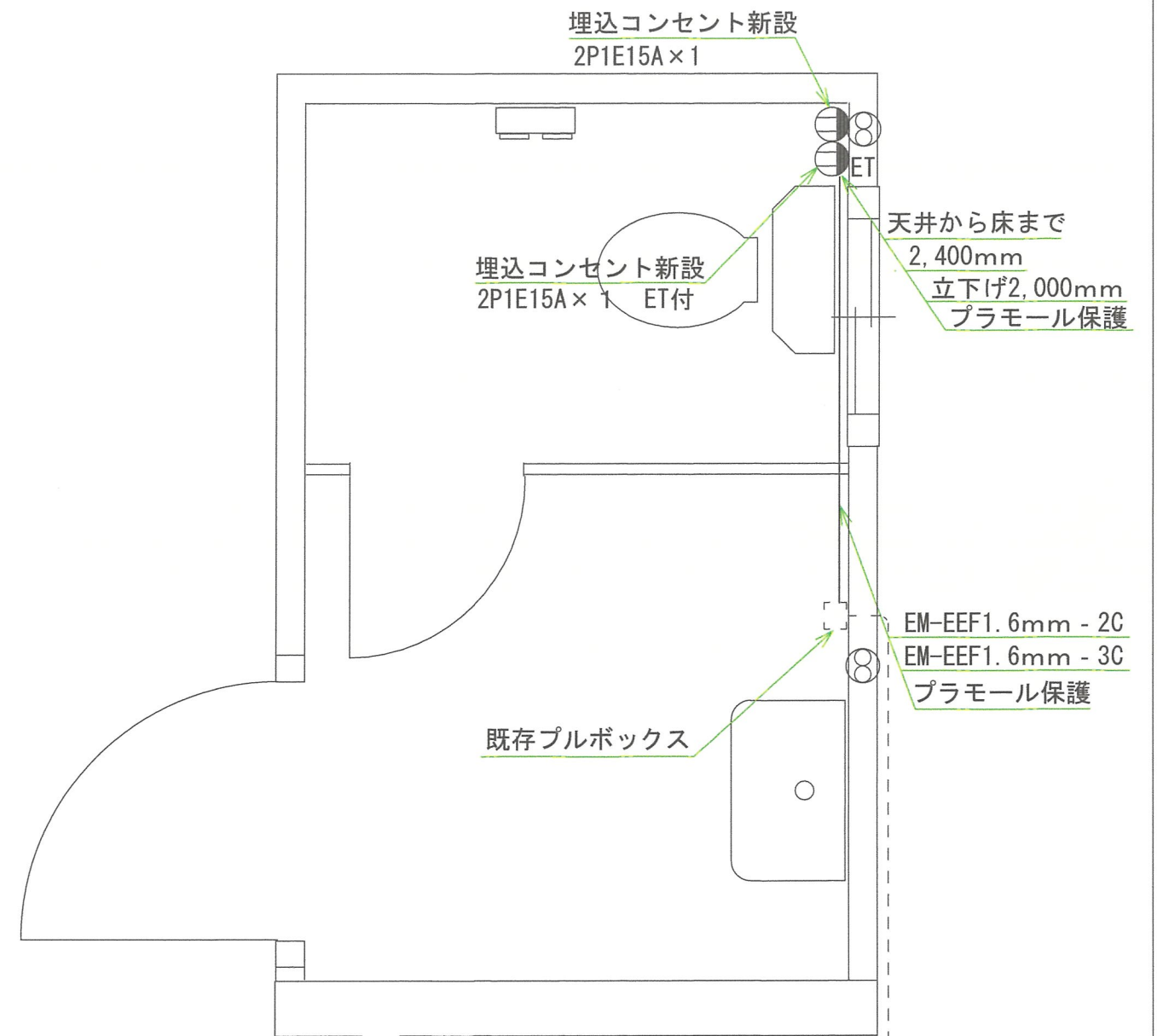
改修後平面図 S=1/20
