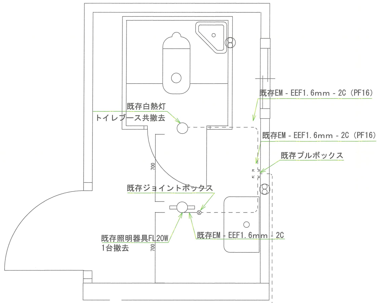
改修前平面図 S=1/20
