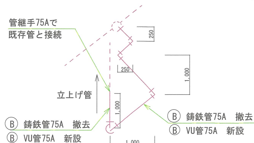
B 通気配管系統図 S=1/X
