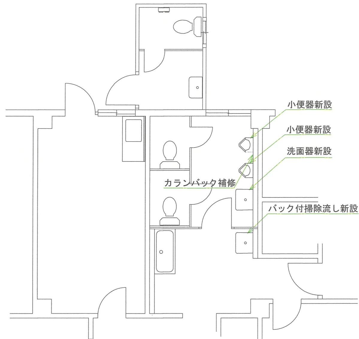
改修後衛生設備平面図 S=1/60
