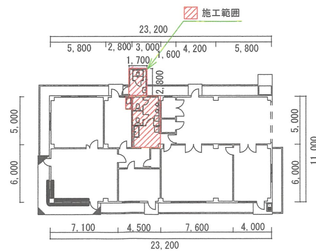
3号警衛所平面図 S=1/400
