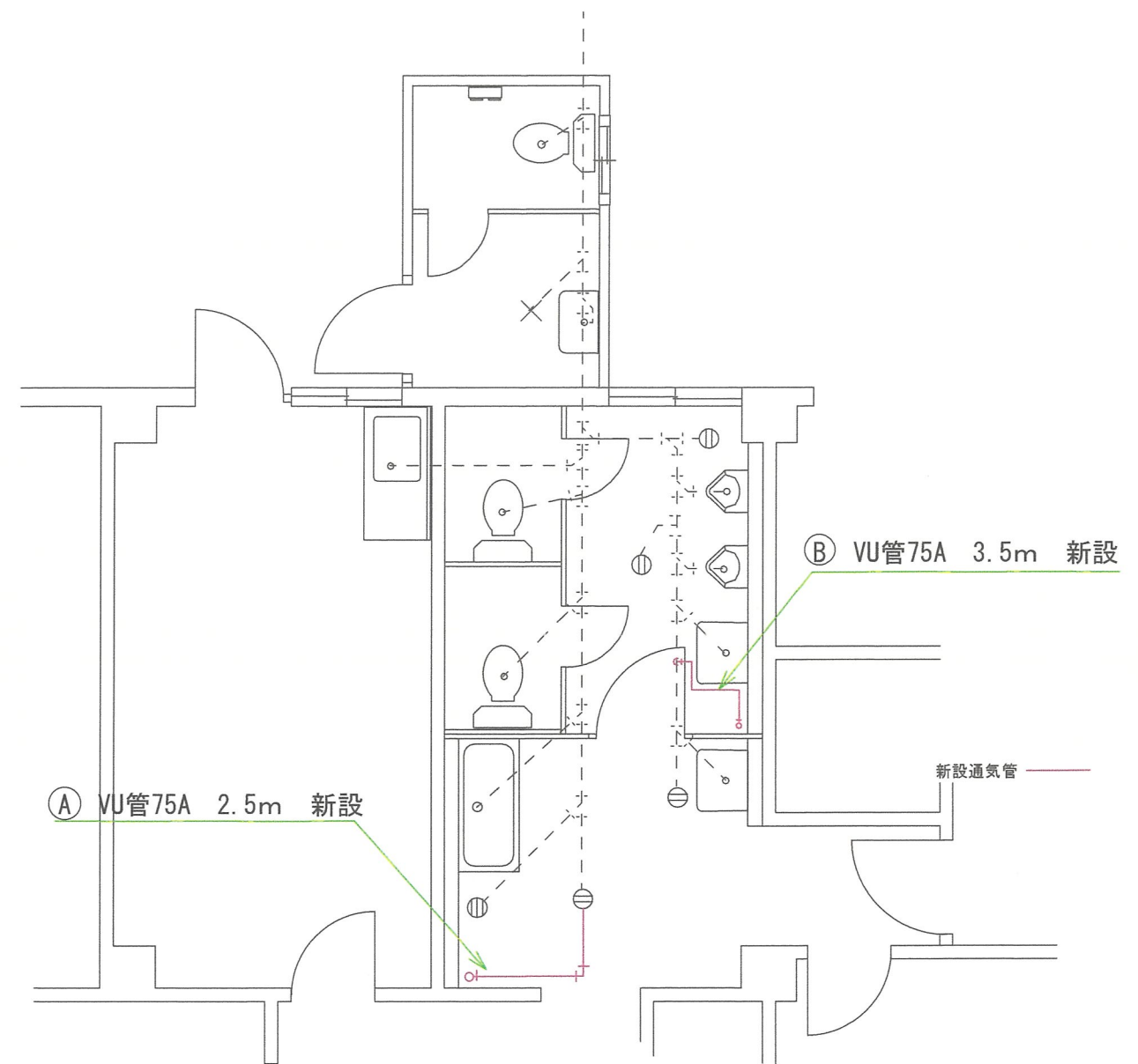
改修後平面図 S=1/60
