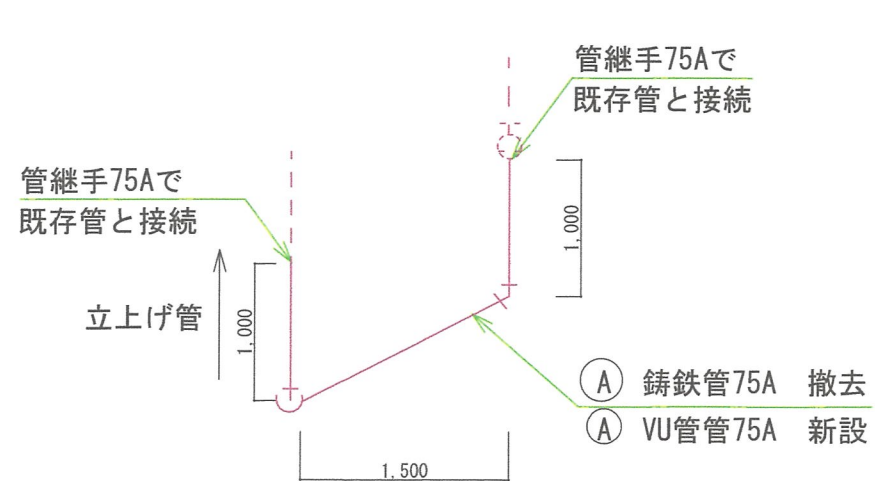
A 通気配管系統図 S=1/X
