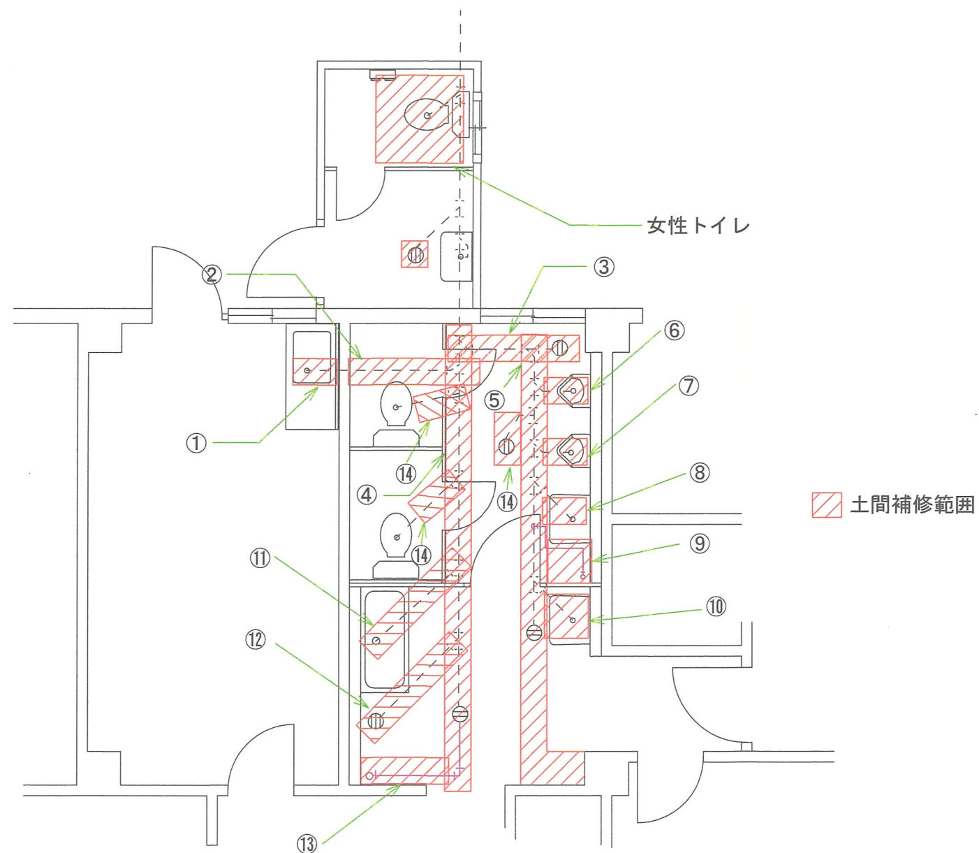
土間補修範囲平面図 S=1/60
