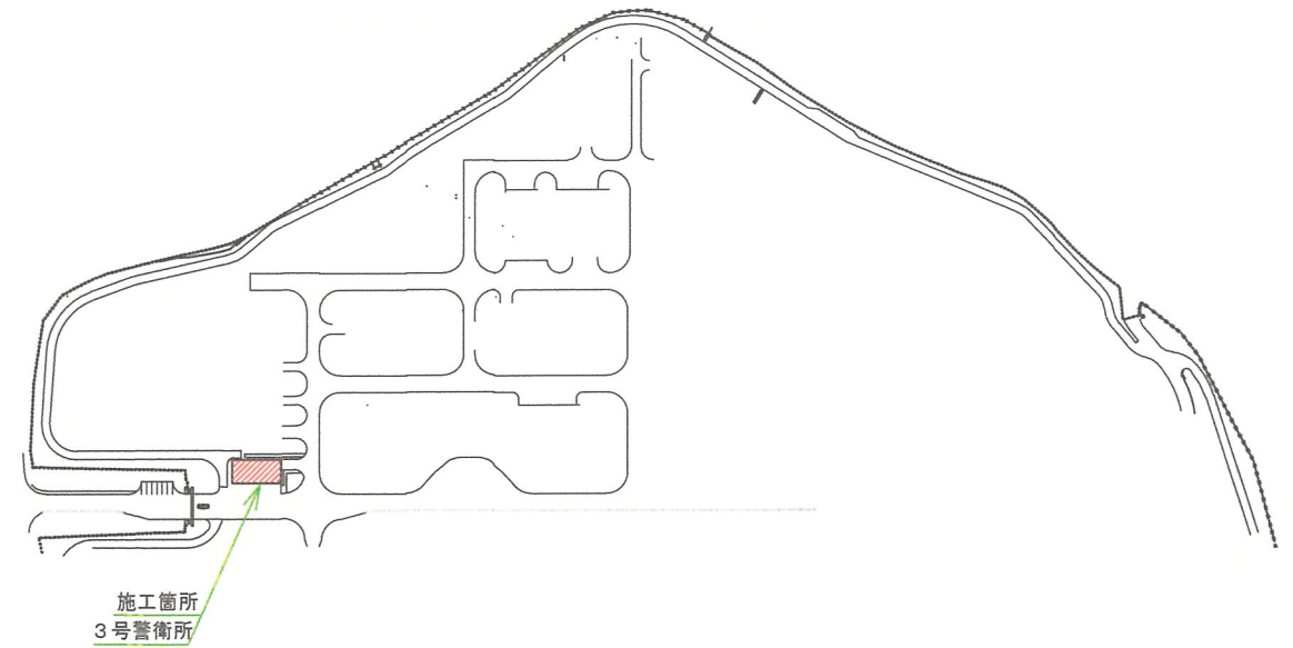
駐屯地配置図 S=1/4,000
