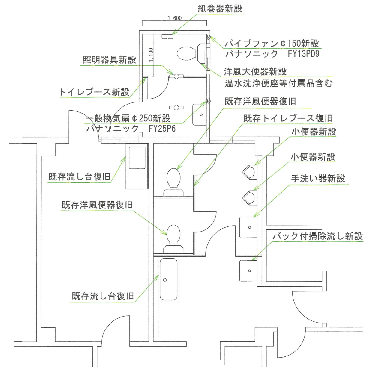
改修後平面図 S=1/60
