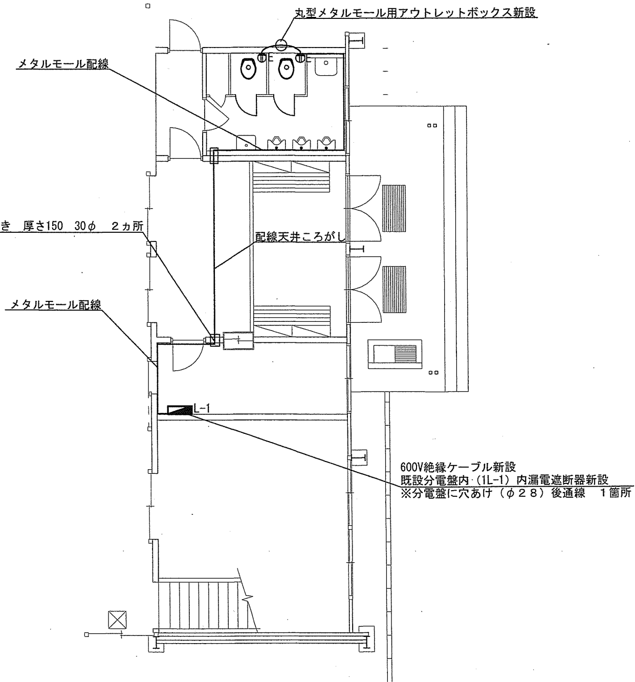
108号建物1階改修電気設備平面図 S=1:100
