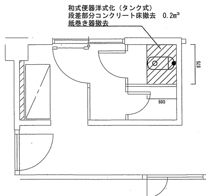
202号建物便所改修前平面図 S=1:50
