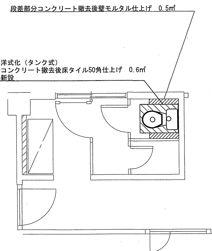
202号建物便所改修後平面図 S=1:50
