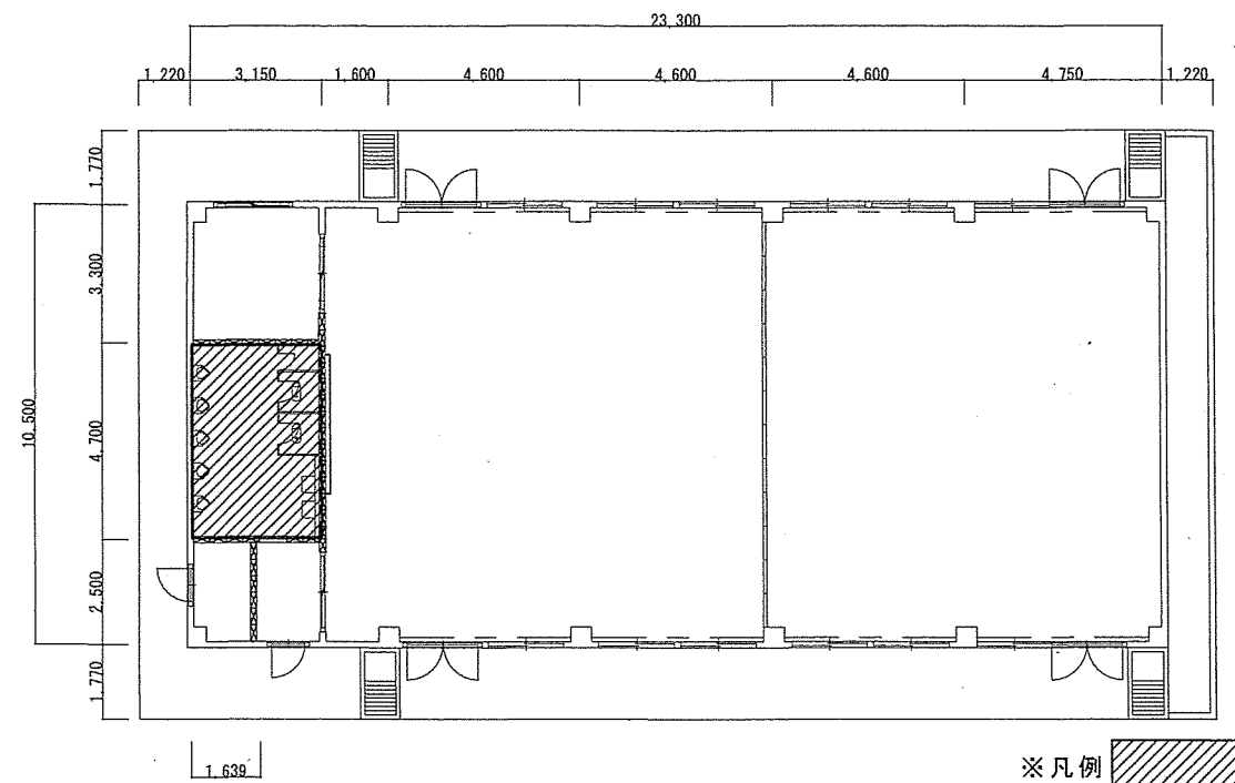
107号建物平面図S=1:200
