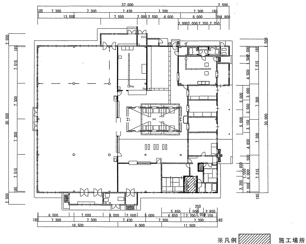
103号建物平面図 S=1:400
