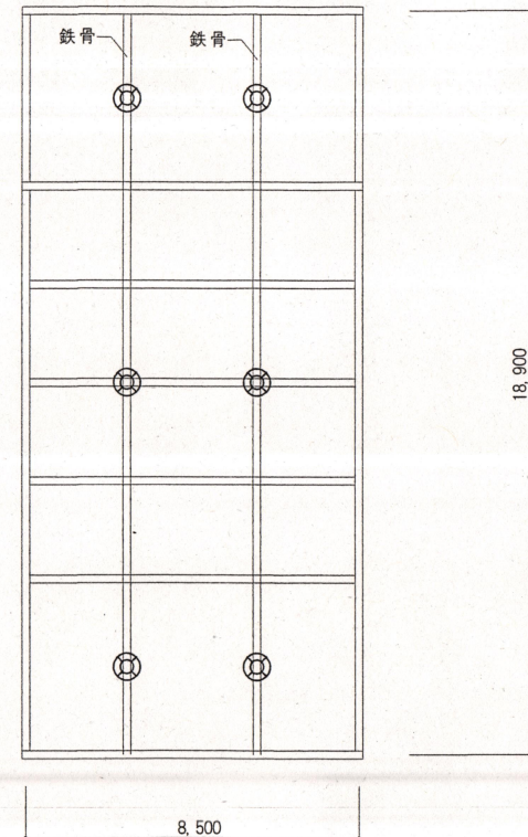
スタンド上屋電灯設備図 S=1:150
