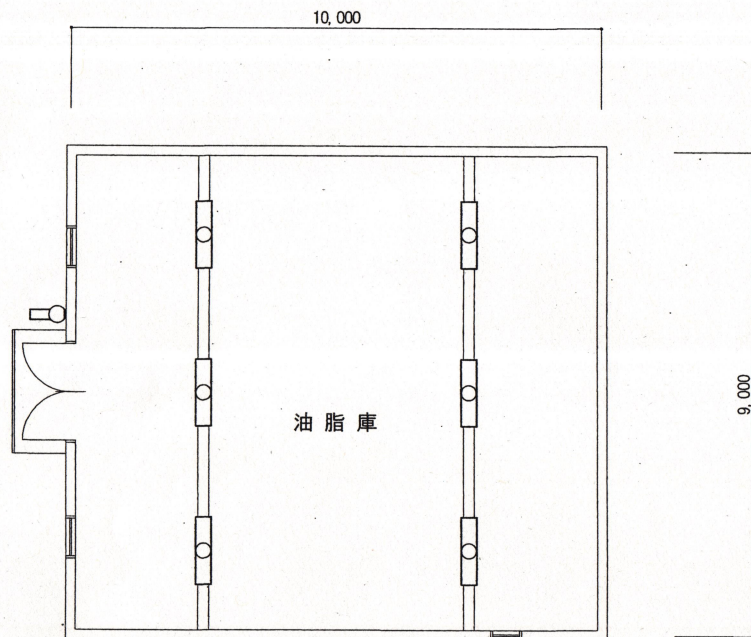
141号建物電灯設備図 S=1:100
